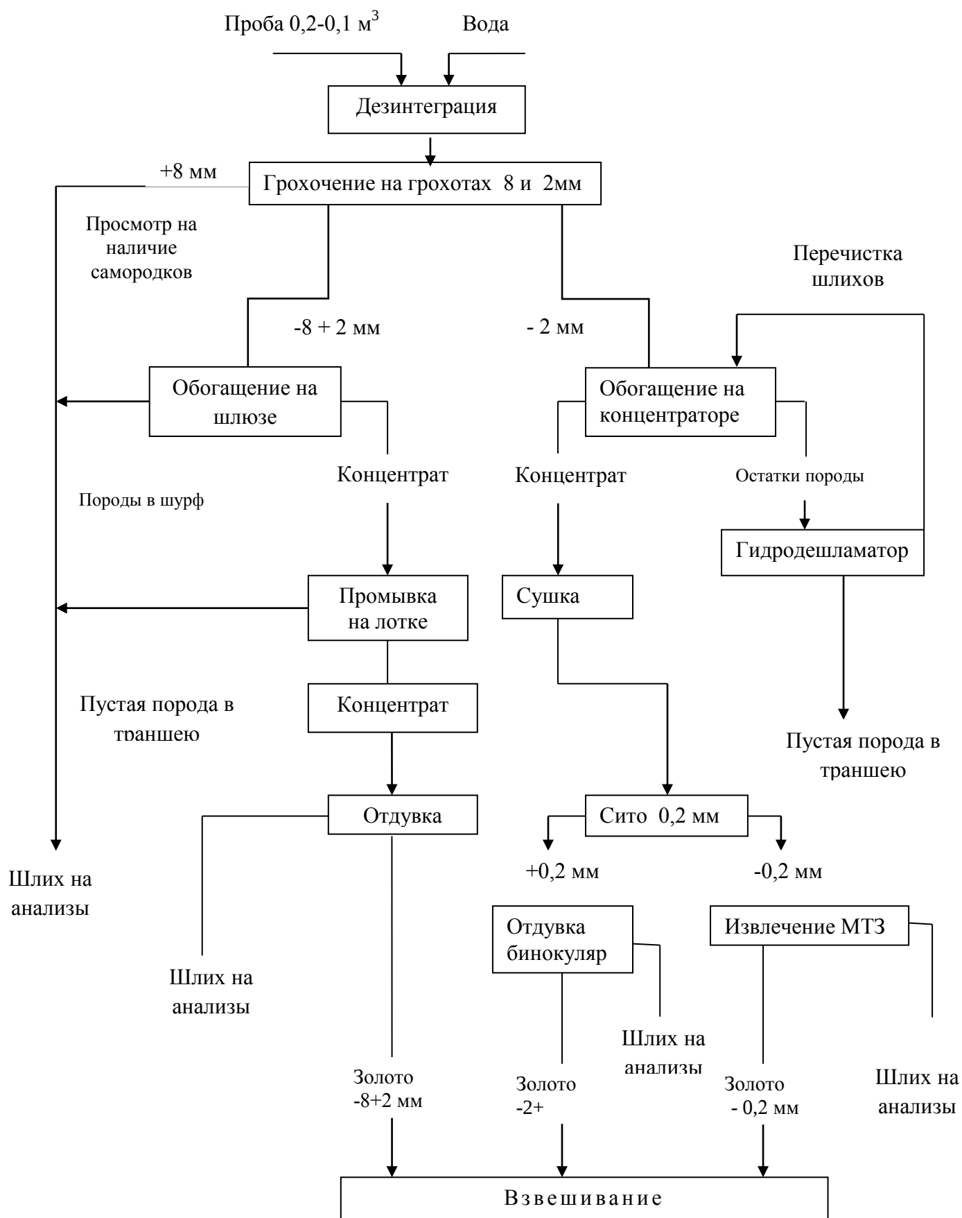
Рис.5 Схема обработки шлиховых проб
