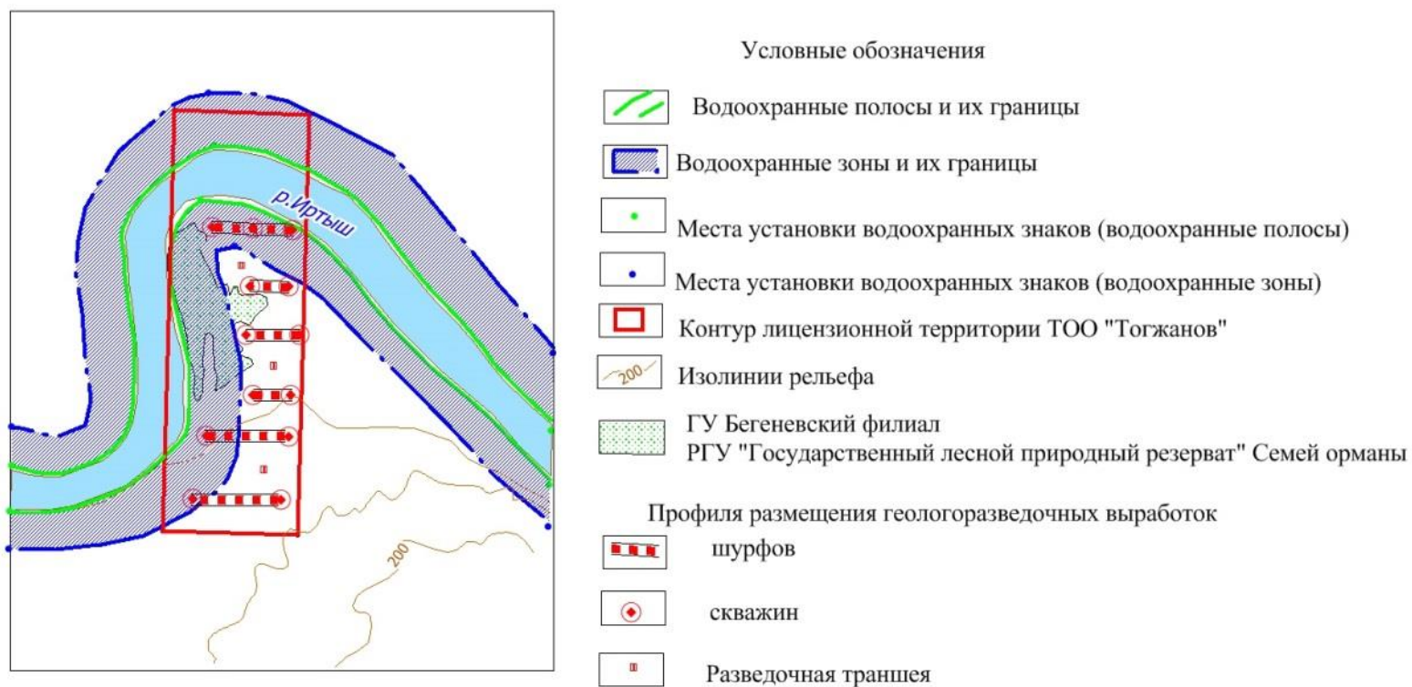
Схема размещения горных выработок Масштаб 1:50 000
