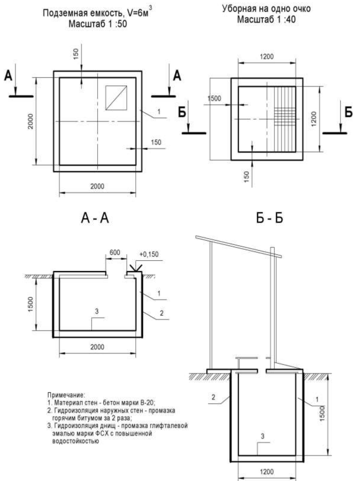
Рис. 6.3 Туалет
