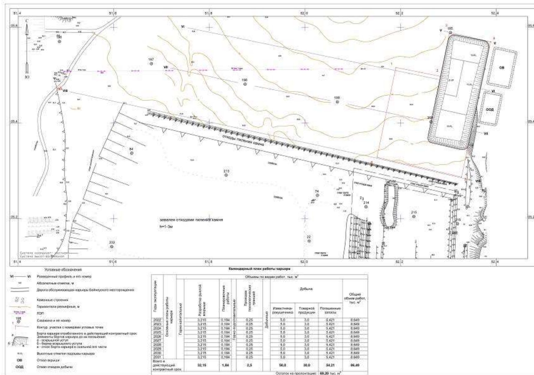
Рис.7. План карьера на конец погашения запасов
