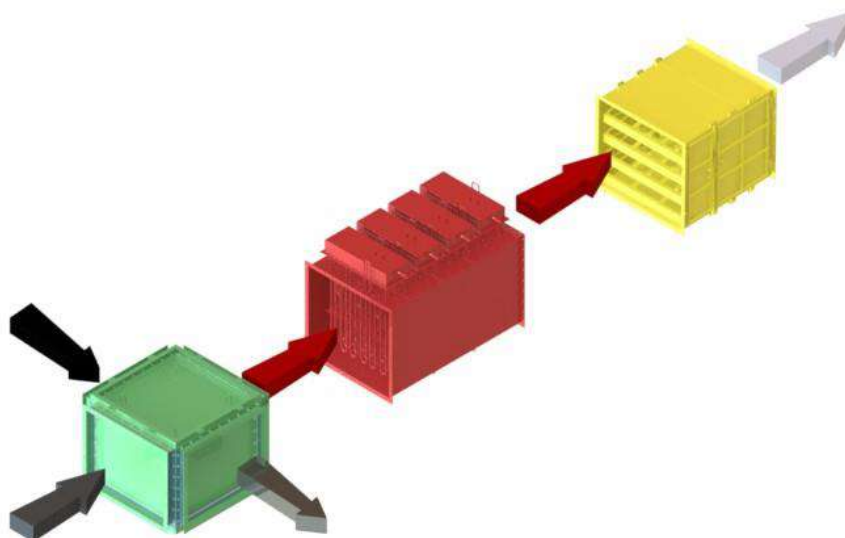
Рисунок 1. Основные принципиальные блоки установки термокаталитической – теплообменник, блок нагрева, реактор.
