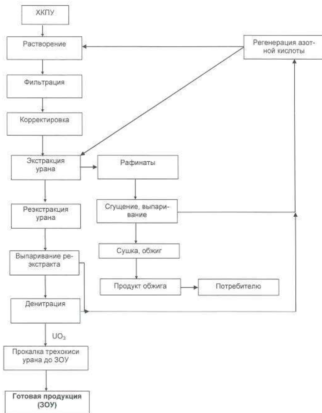
Рис. 3.1.3 Принципиальная схема изготовления порошка U_3O_8 с использованием технологии канадской компании Сатесо.
