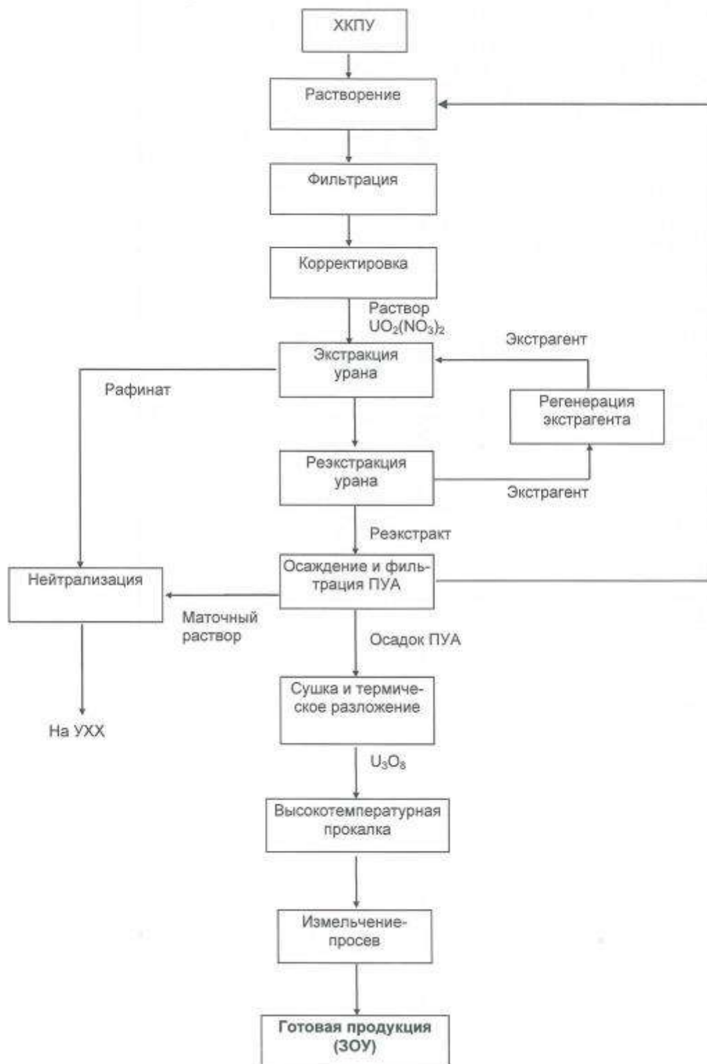
Рис. 3.1.2 – Схема технологического процесса переработки ХКПУ (существующая).
