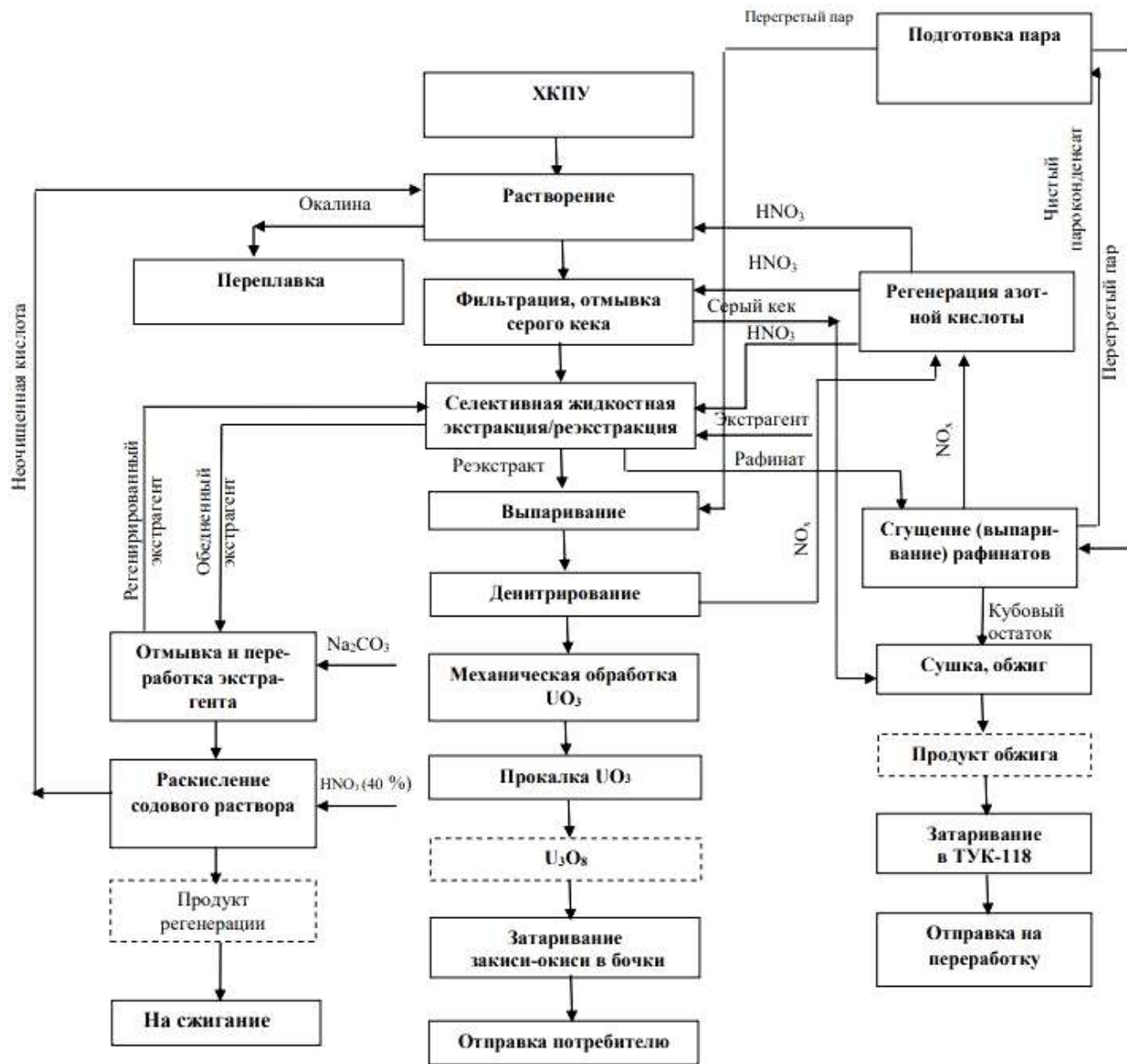
Рис. 1 - Принципиальная схема производства.
