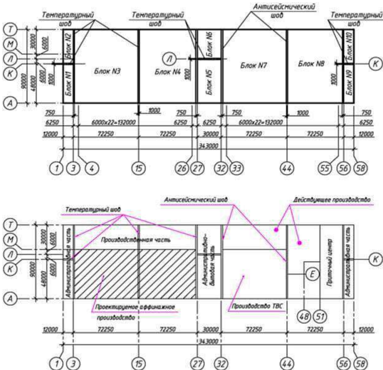
Рисунок 4.4 – Разделение здания 600 на блоки (штриховкой выделен участок аффинажного производства)
