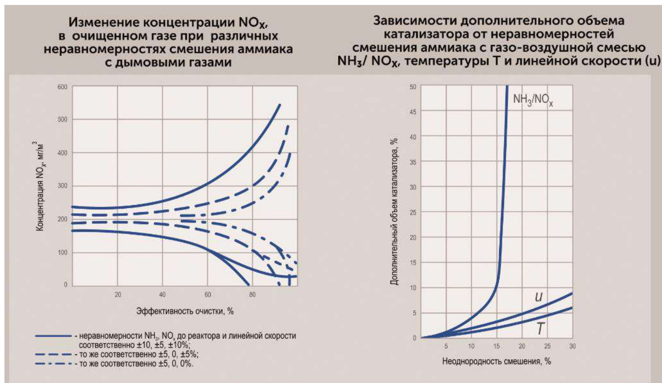
Рисунок 3 – Зависимости изменения концентраций \text{NO}_x
