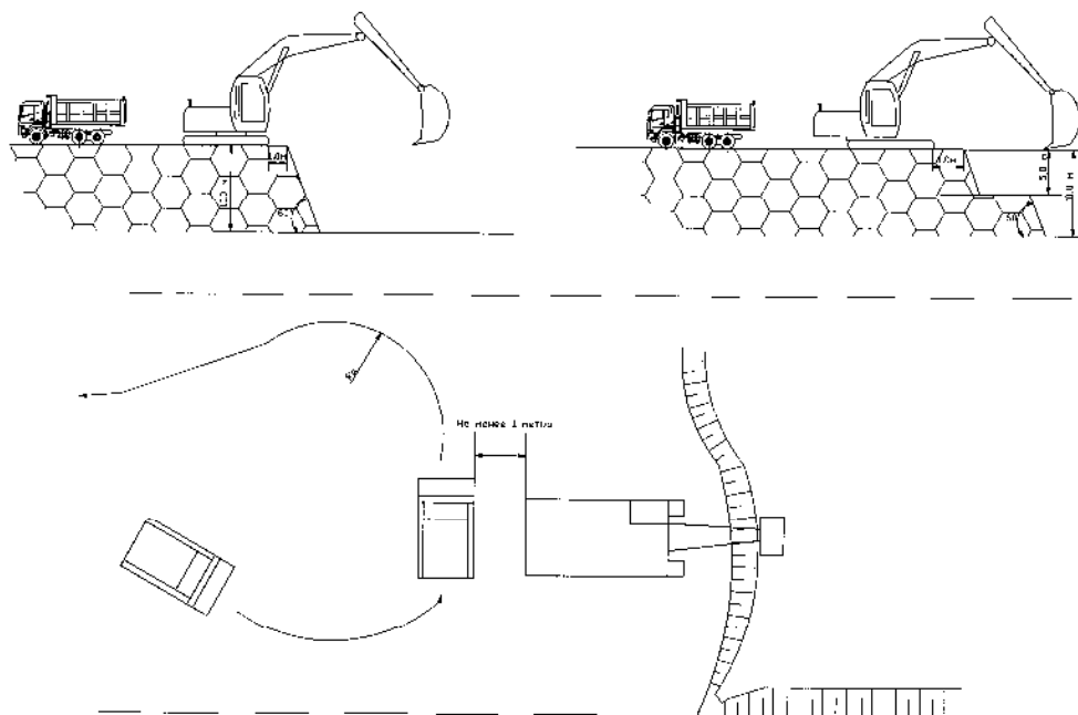
Рис.2. Технологическая схема отработки уступа с верхней погрузкой
