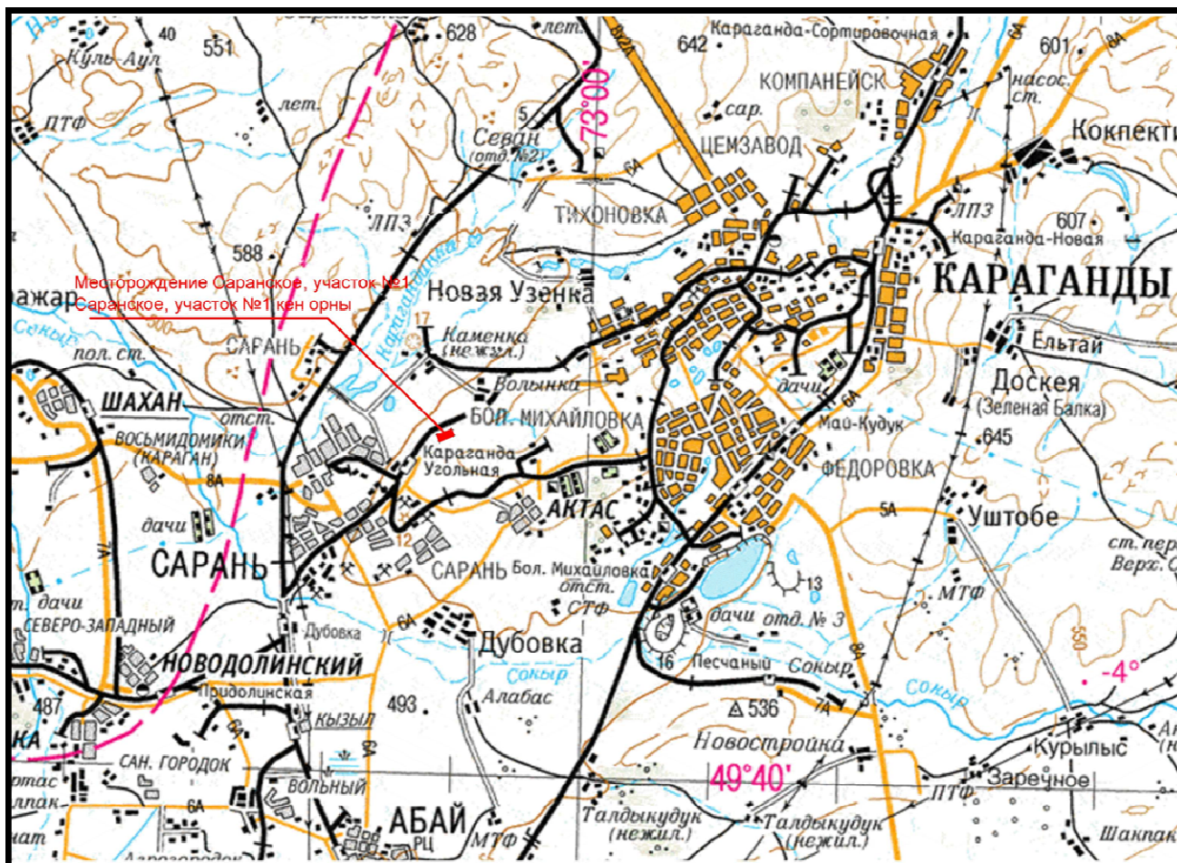
Ситуационная (обзорная) схема
