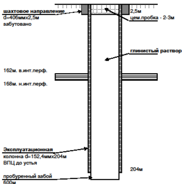
Фактическая схема конструкции скважины до ликвидации
