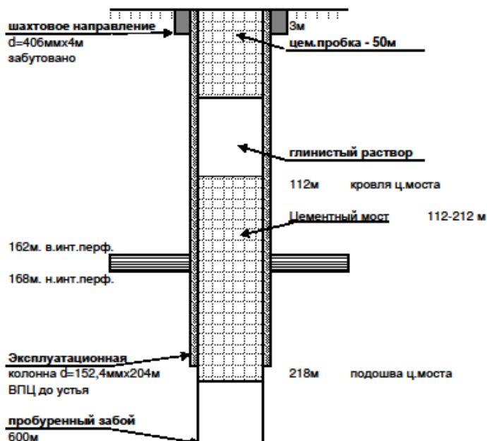
Рисунок 4.4.1– Конструкция скважины Чиили 2
