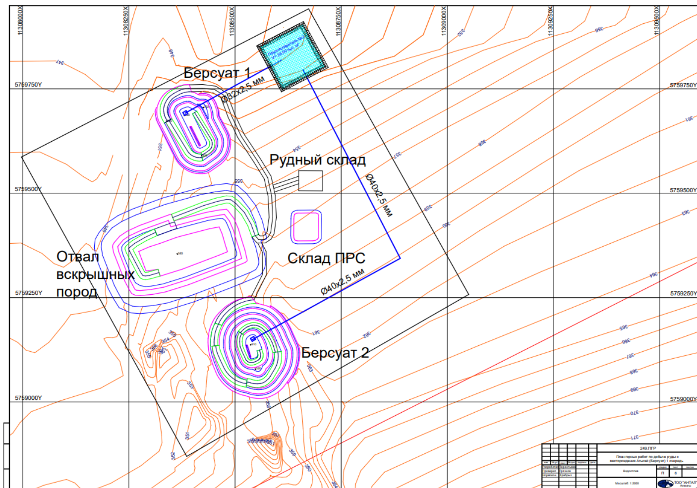
Рис. 2.1 – Генеральный план месторождения
