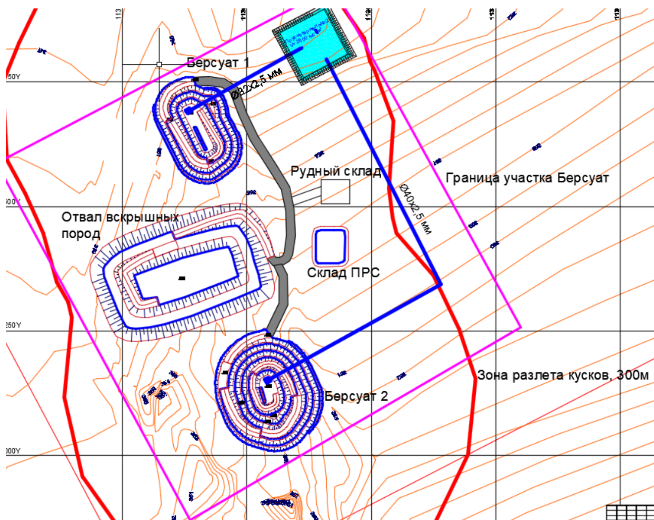
Рис. 1.4.1 - Ситуационный план месторождения М 1:2 000
