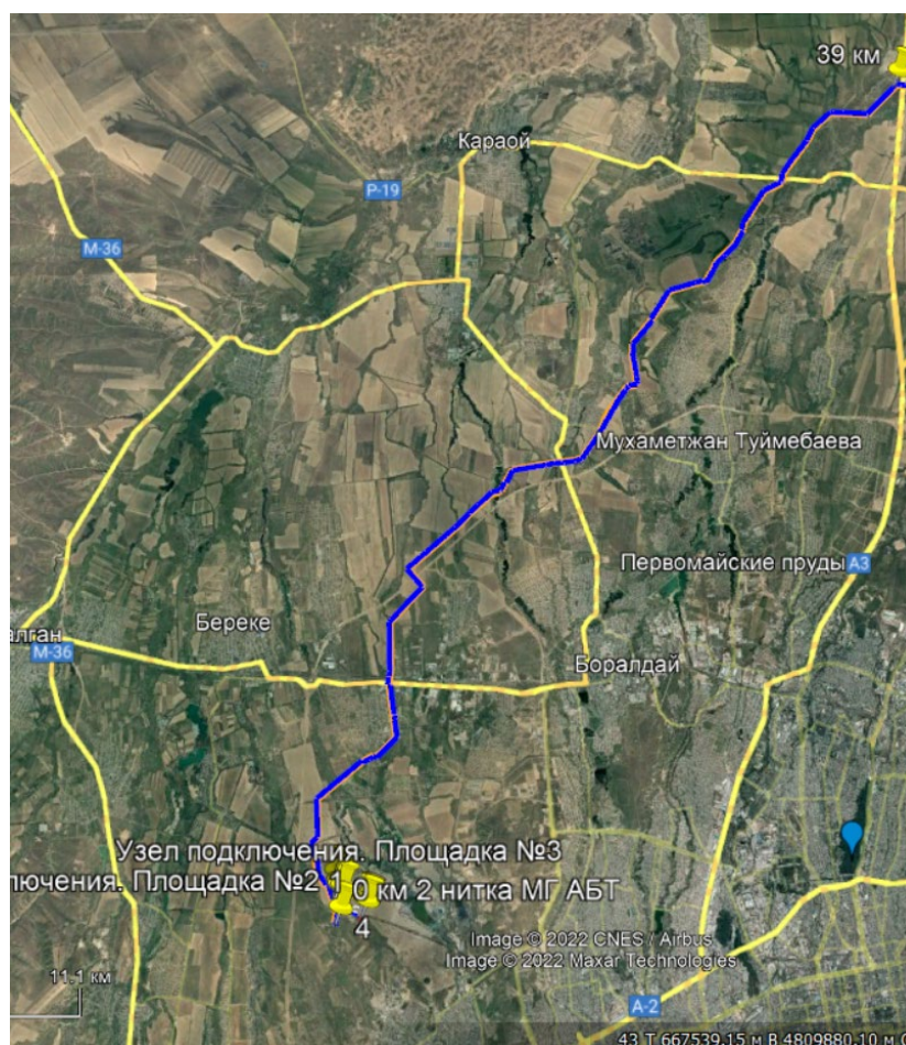
Рис. 1 Ситуационная схема размещения проектируемого объекта
