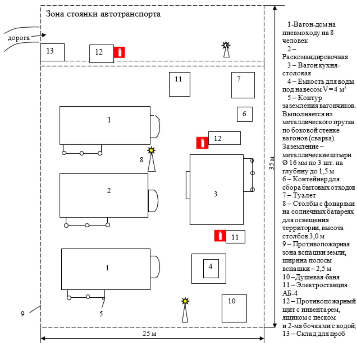
Рисунок 3 – Предполагаемая схема размещения полевого лагеря
