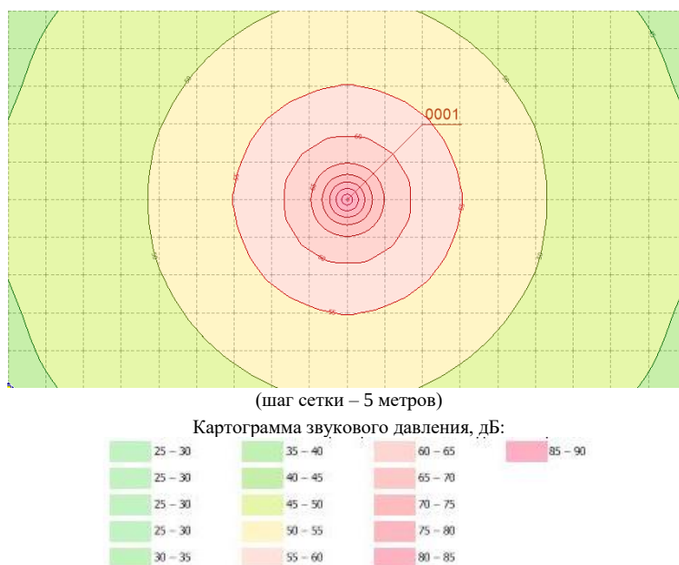
Рисунок 4 – Результаты расчёта затухания звука в графической форме в рабочей зоне оборудования при проведении разведочных работ (эквивалентный уровень звука – интегральный показатель)
