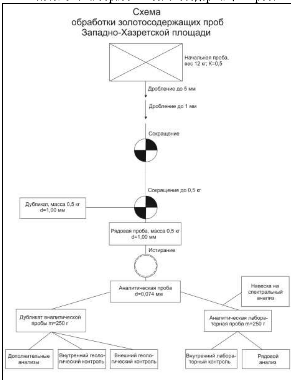
Рис.5.6. Схема обработки золотосодержащих проб.
