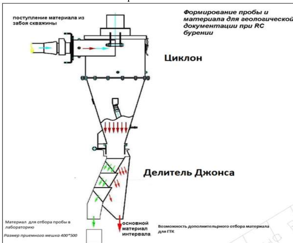
Рис.5.5. Схема расположения оборудования для отбора шлама/пробы из скважины RC.
