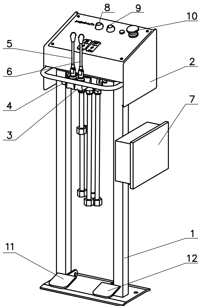
Рисунок 7. Пульт управления.
