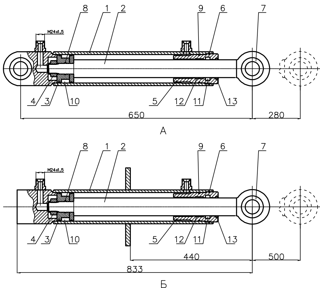
Рисунок 11. Гидроцилиндр.
