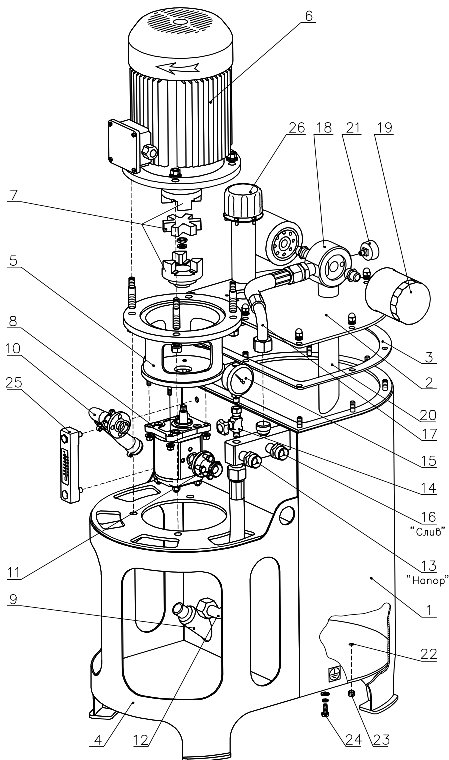
Рисунок 9. Установка насосная.
