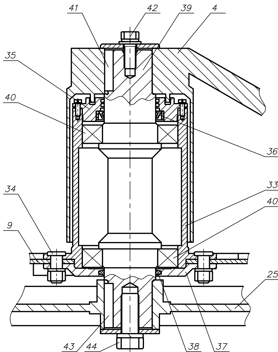
Рисунок 4. Опора ротора.
