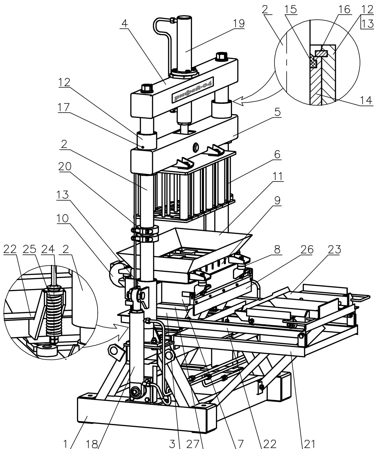
Рисунок 6. Вибропресс.
