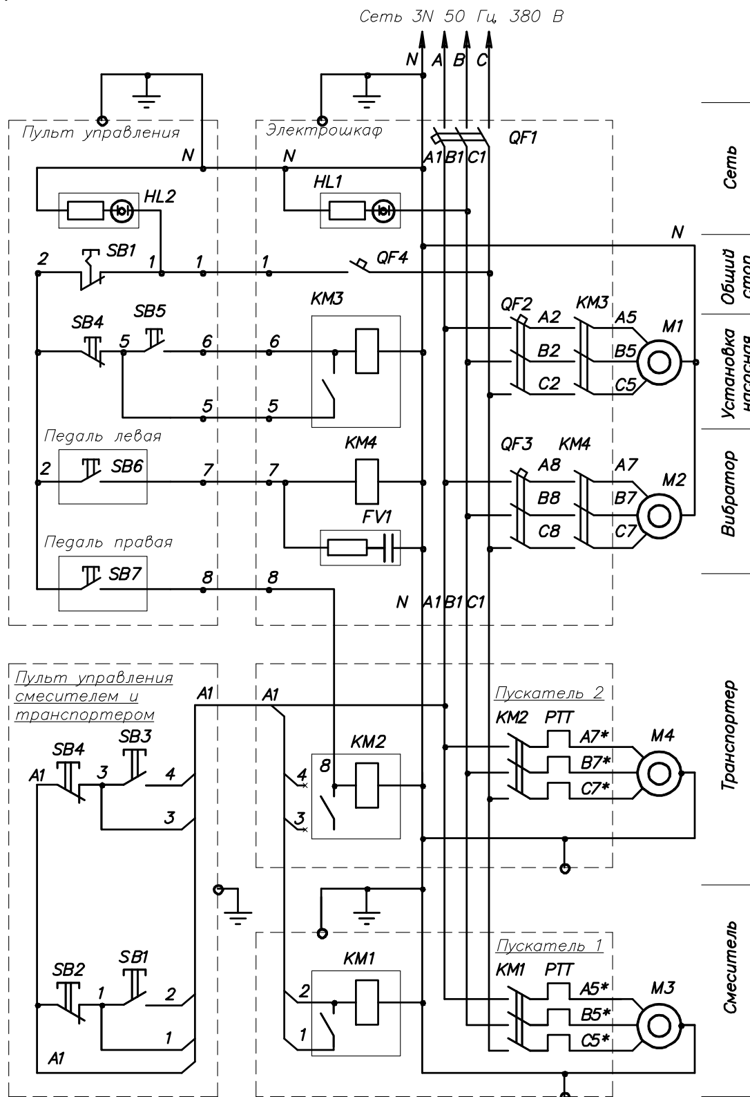
Рисунок 12. Схема электрическая принципиальная.
