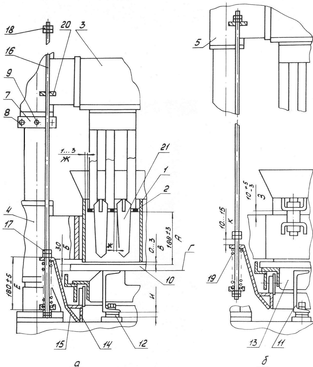
Рисунок 15. Схема контроля высоты стенового камня и настройки рельсового пути.
