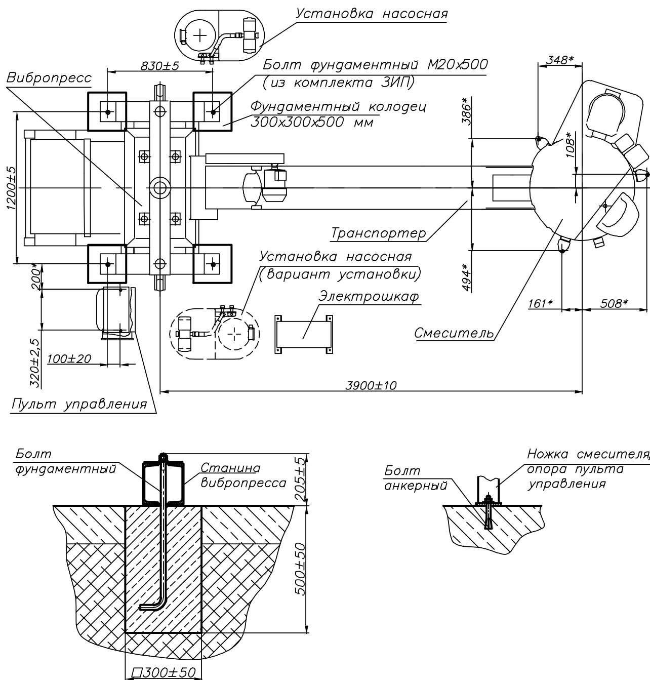
Рисунок 14. План фундамента.
