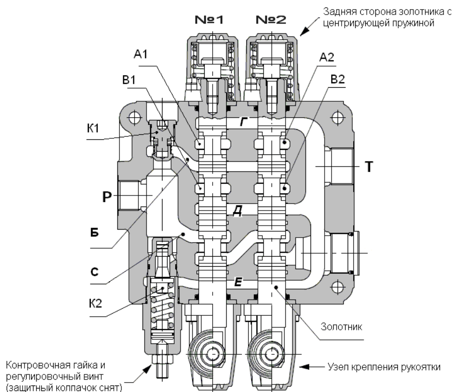
Рисунок 10. Гидрораспределитель НС-D10/2.
