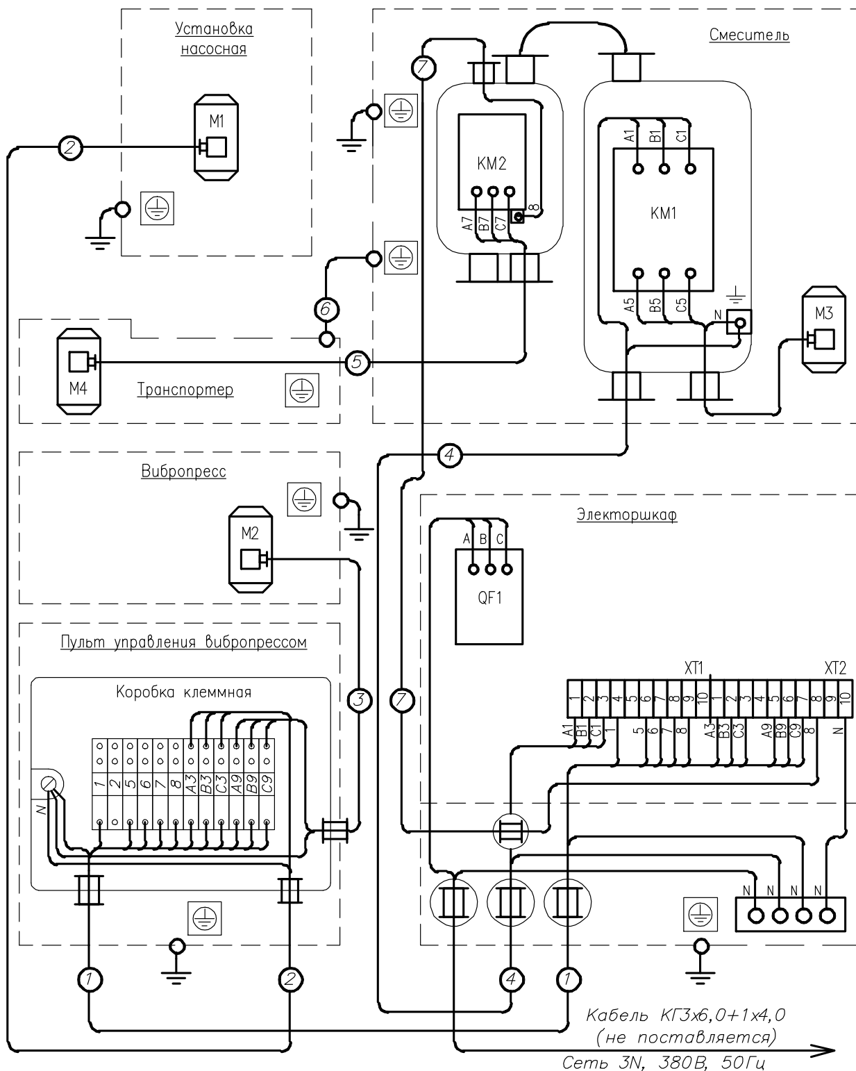
Рисунок 13. Схема электрическая подключения.
