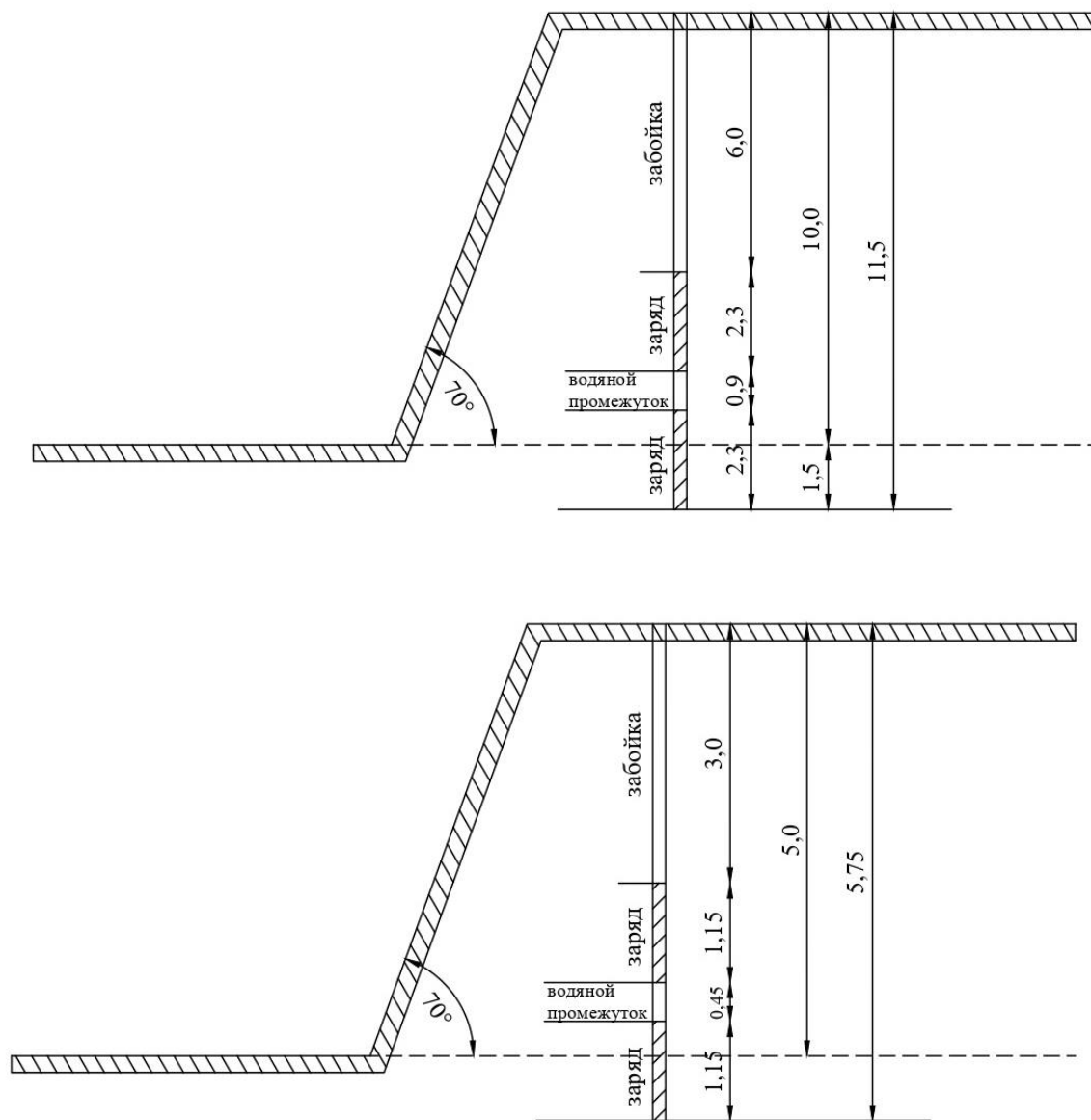
Рисунок 4.3. Схема скважинного заряда.
