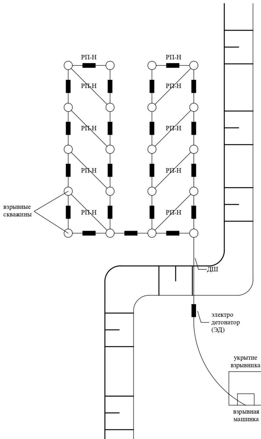
Рисунок 4.4. Схема монтажа взрывных сетей при производстве буровзрывных работ
