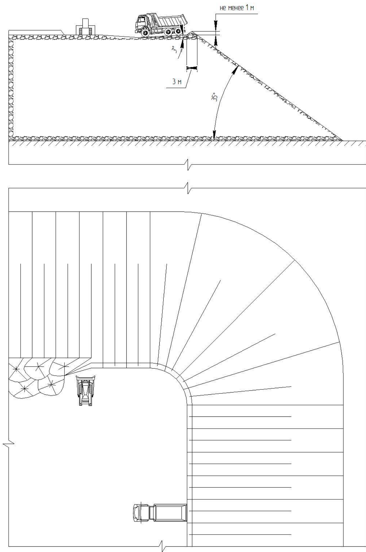
Рисунок 4.5. Схема отвалообразования.
