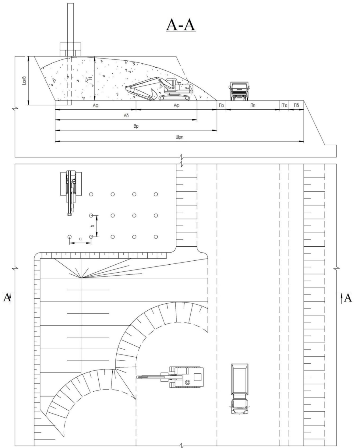
Рисунок 4.2. Параметры рабочей площадки при отработке уступа (подступа) экскаватором с погрузкой в автосамосвал
