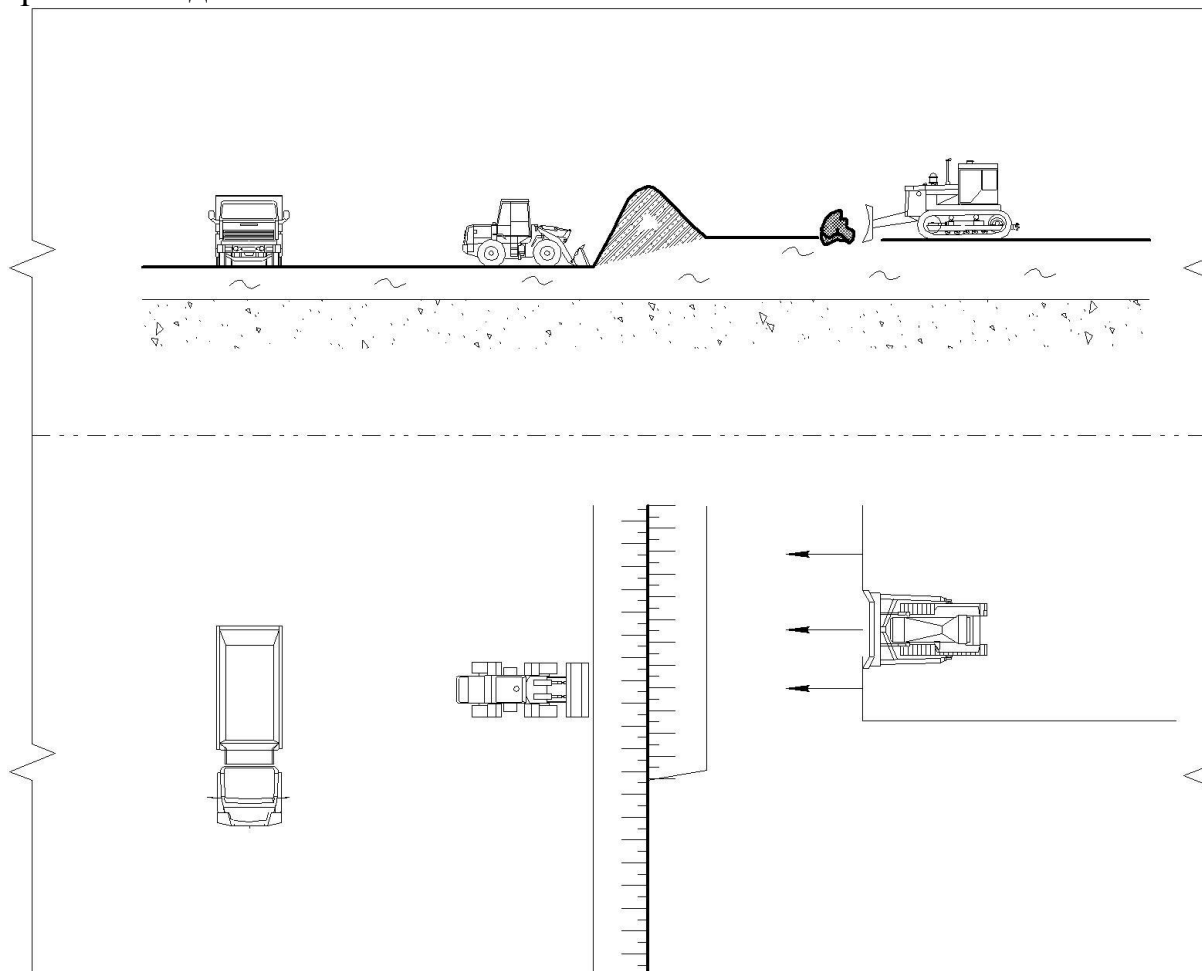
Рисунок 4.1. Схема снятия почвенно-растительного слоя
