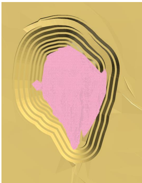
Рисунок 2.1 Контур карьера на конец отработки
