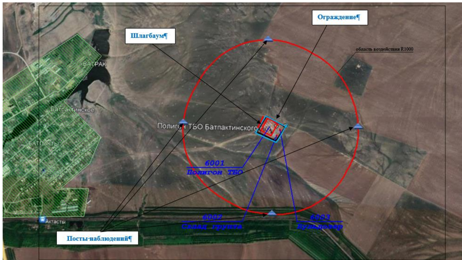
Рисунок 4.2 - Карта-схема расположения источников загрязнения и СЗЗ предприятия
