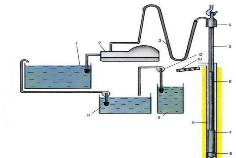
Рис.11 Схема оборотного водоснабжения
