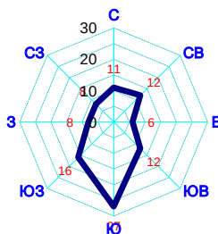
Рис.1.1. Роза ветров.
