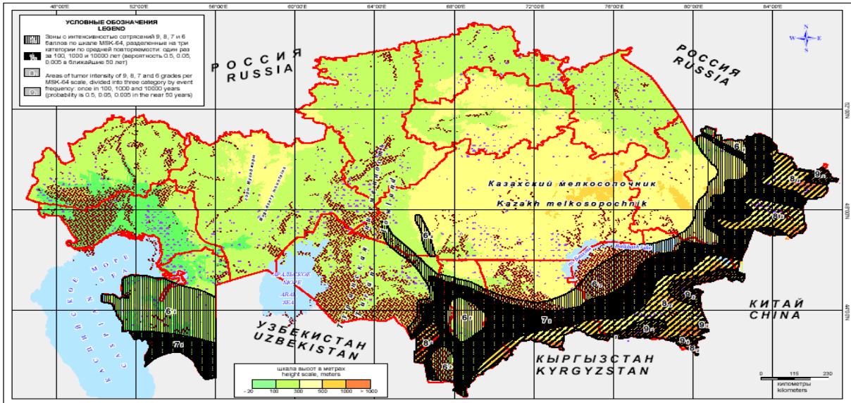
Рисунок 2.4- Карта сейсмического районирования Республики Казахстан
