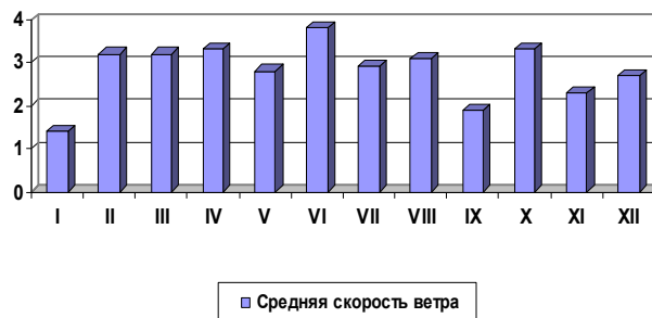
Рисунок 6 - Средняя месячная скорость ветра (м/с)
