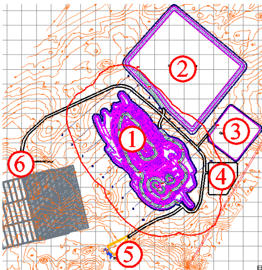
Рис. 2.1 – Генеральный план месторождения
