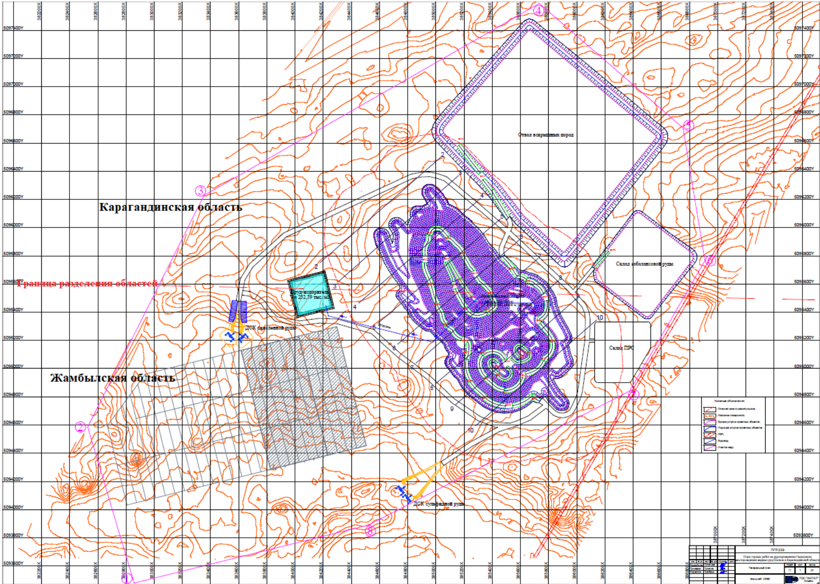
Рис. 1.4.1 - Ситуационный план месторождения
