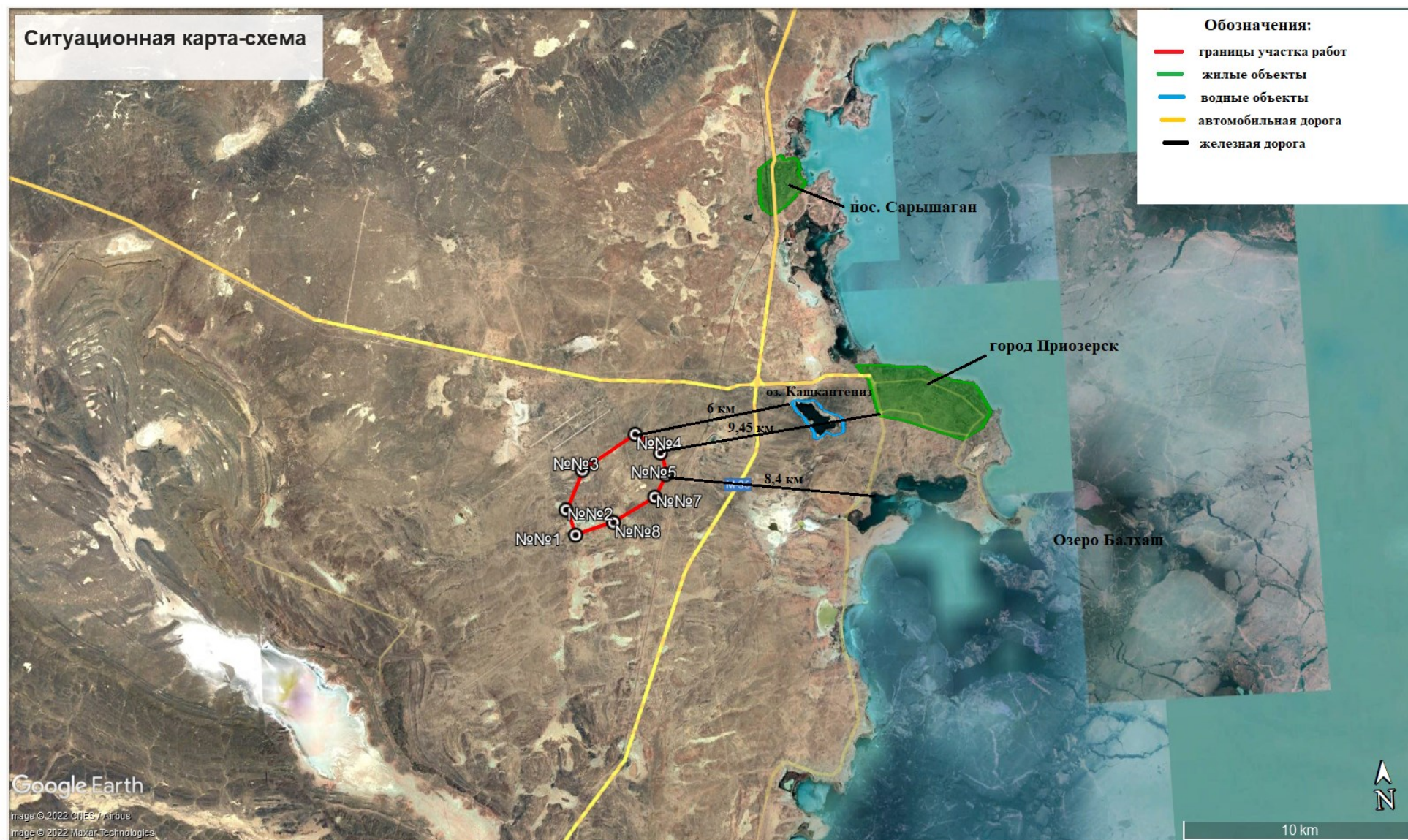
Рис. 1.2 – Ситуационная карта-схема площадки размещения месторождения
