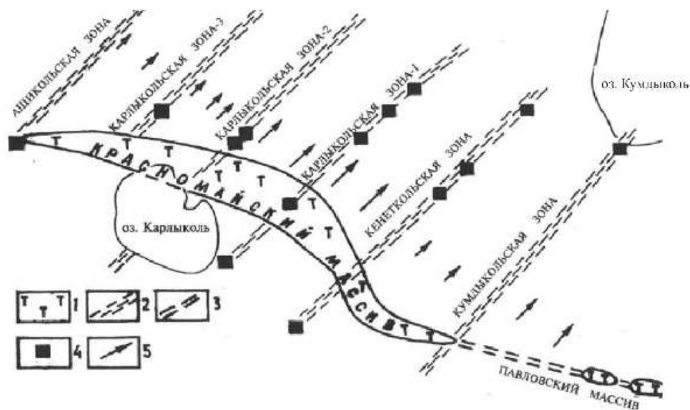
ДИНАМИЧЕСКАЯ СХЕМА РАЗВИТИЯ КРАСНОМАЙСКОЙ ЗОНЫ. ПО В.Е. Гонтаренко). 1 -пироксениты красномайского комплекса; 2 - зоны углеродной мантийной дегазации; 3 - Красномайский глубокий разлом; 4 - установленная алмазная минерализация; 5 - векторы направления перемещения блоков (длина вектора указывает на скорость передвижения блоков).
