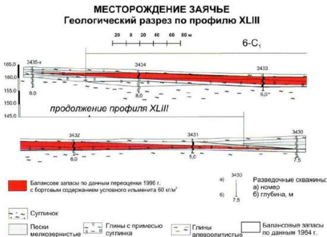
Рисунок 5.2 Геологический разрез на месторождении Заячье
