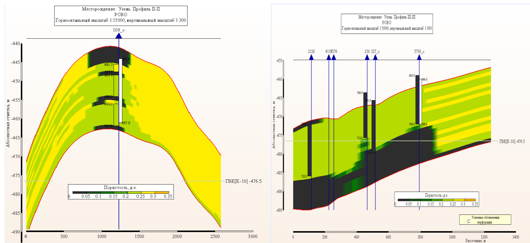
Рисунок 4.3.- Геологические профили распределения пористости пород X газового горизонта по скважинам №№109 и 2126, 4118, 7576, 5730.
