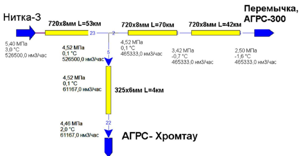
Рисунок 2.4.2.1 □ Схема к гидравлическому расчету 3-нитки газопровода-отвода на г.Актобе
