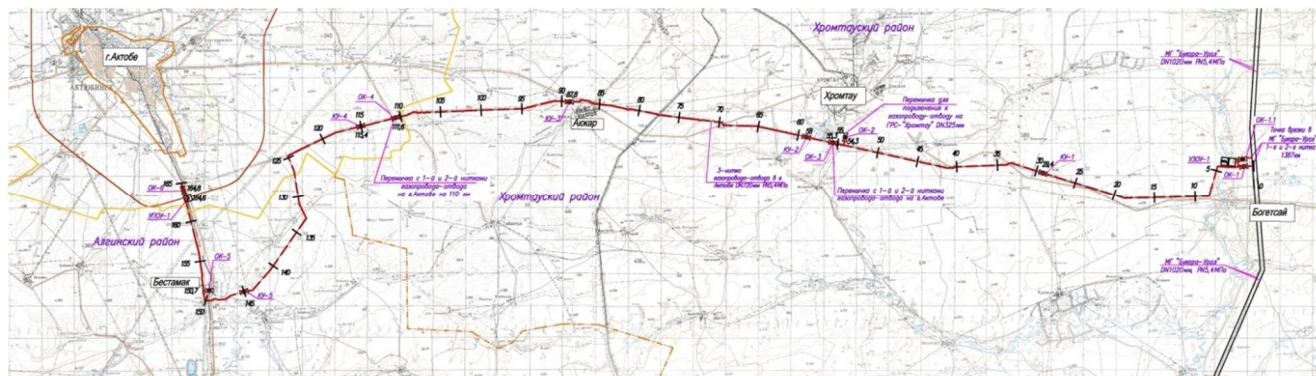
Рисунок 2.2.1 □ Схема трассы 3-нитки газопровода-отвода на г.Актобе
