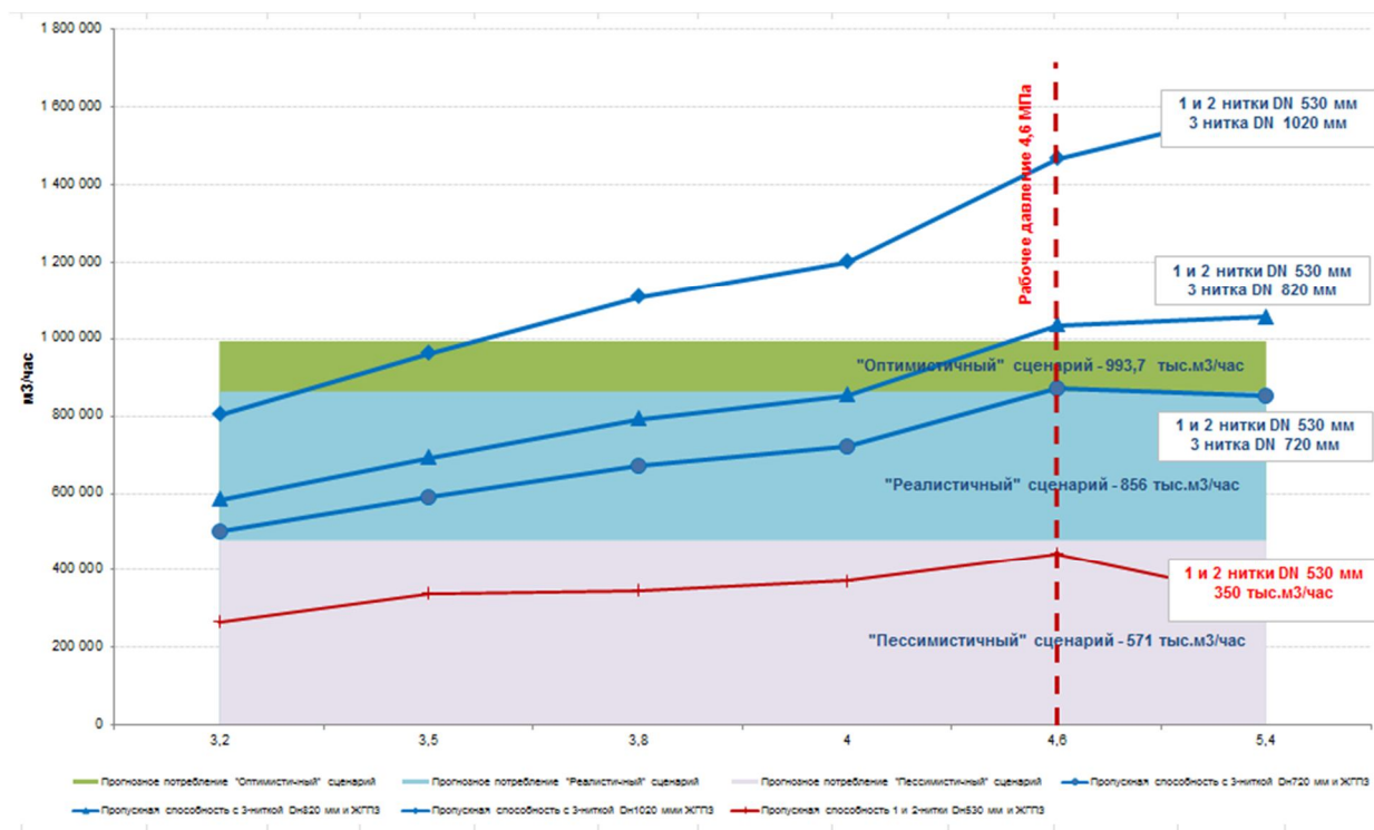
Рисунок 3.1.6.1 □ Результаты гидравлических расчетов газотранспортной системы 1,2 и 3 □ нитки (ТЭО)
