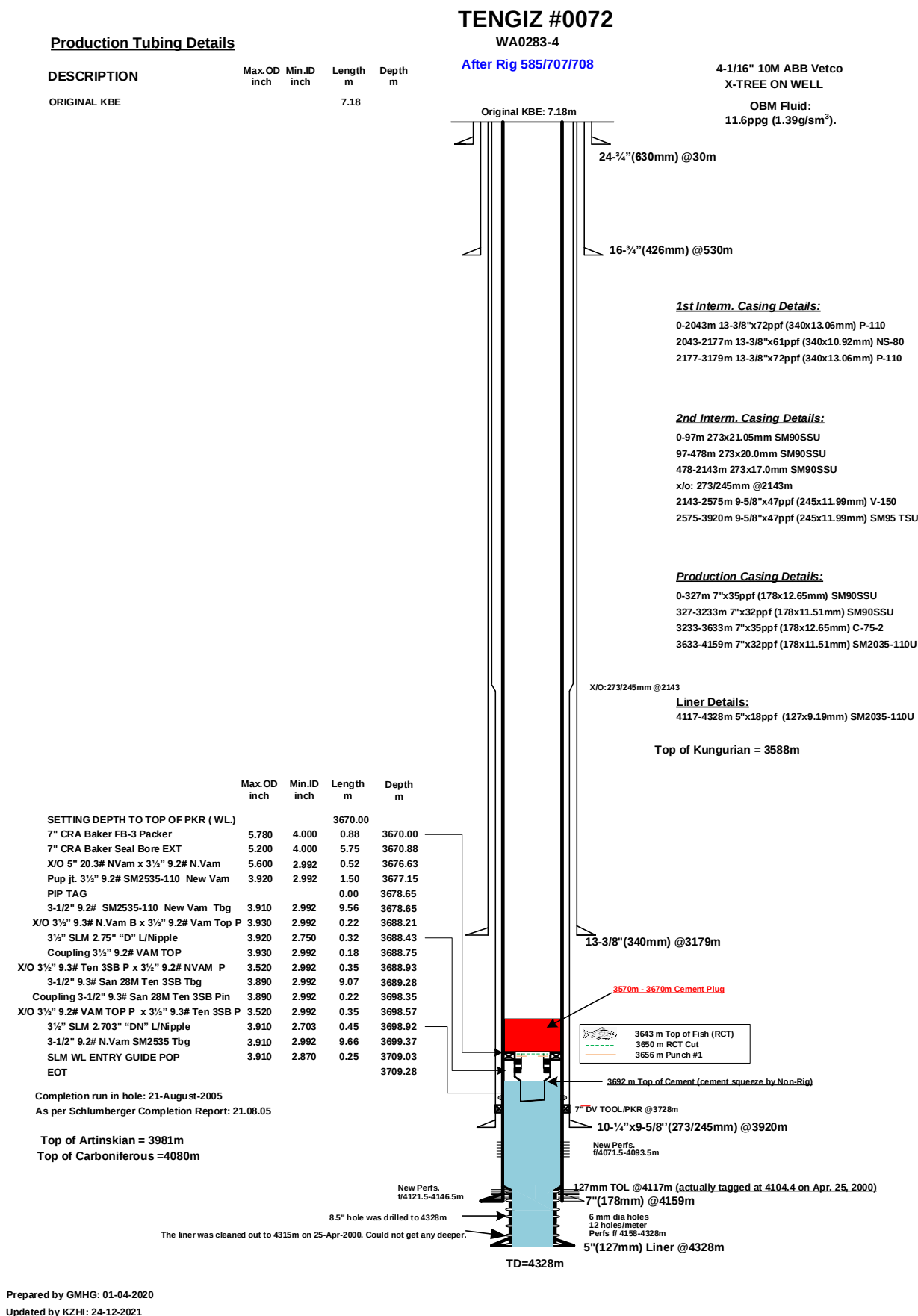
Рисунок 6. Предлагаемая конструкция по завершению изоляционно-ликвидационных работ по скважине Т-0072
