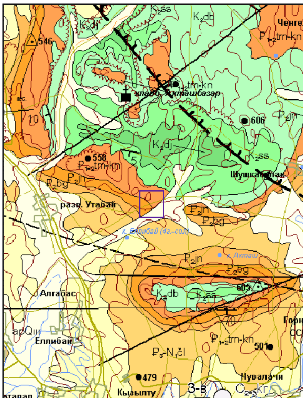
Рис. 2 Геологическая карта участка
