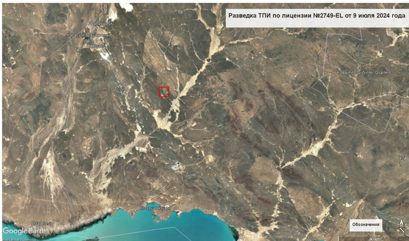
Космоснимок района работ
