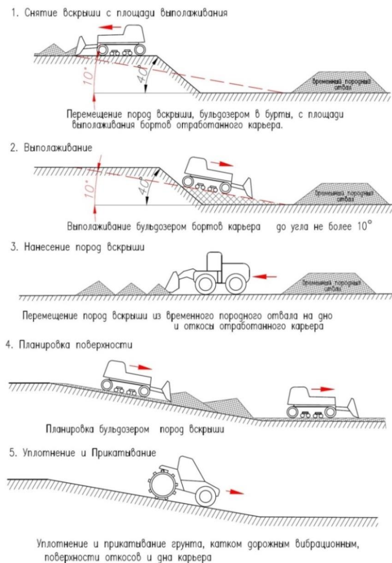
Рис.7.3.2 Принципиальная схема рекультивации
