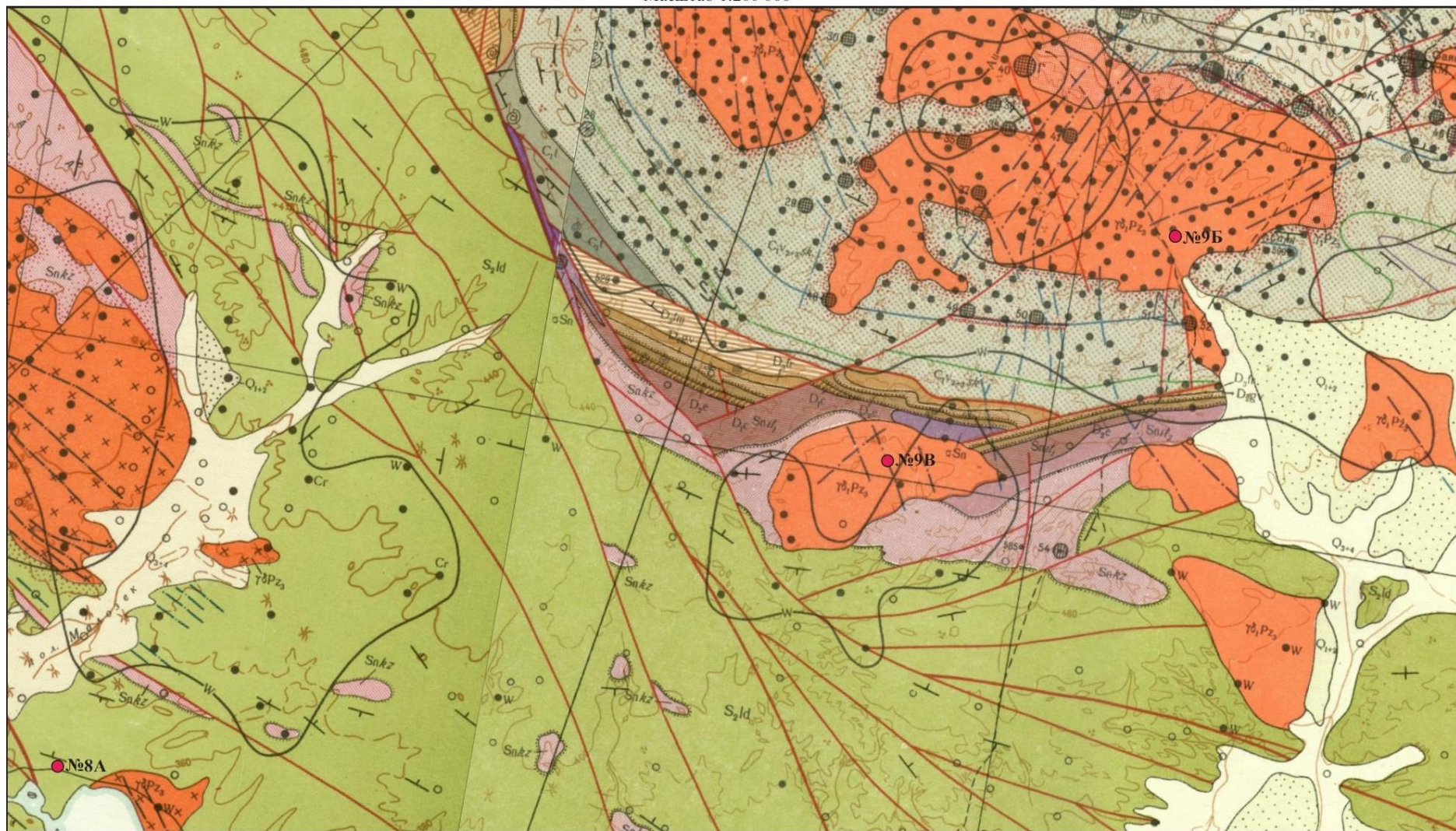
Рис.2.2 Геологическая карта расположения участков №8А, №9В, №9Б. Масштаб 1:200 000
