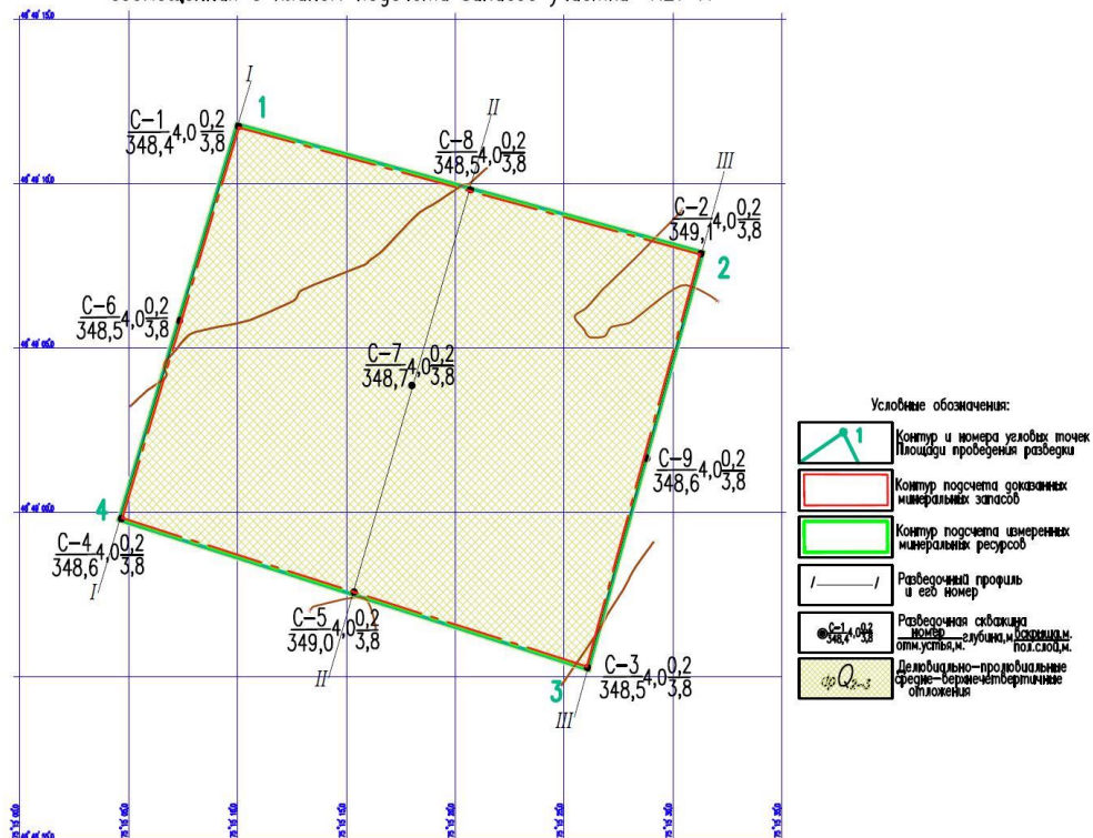
Геологическая карта совмещенная с планом подсчета запасов участка "N27 А"
