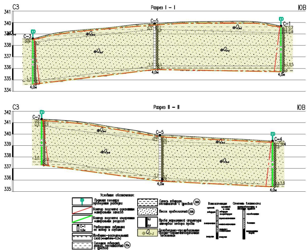
Рис. 2.5 Схема геологического строения участка №28
