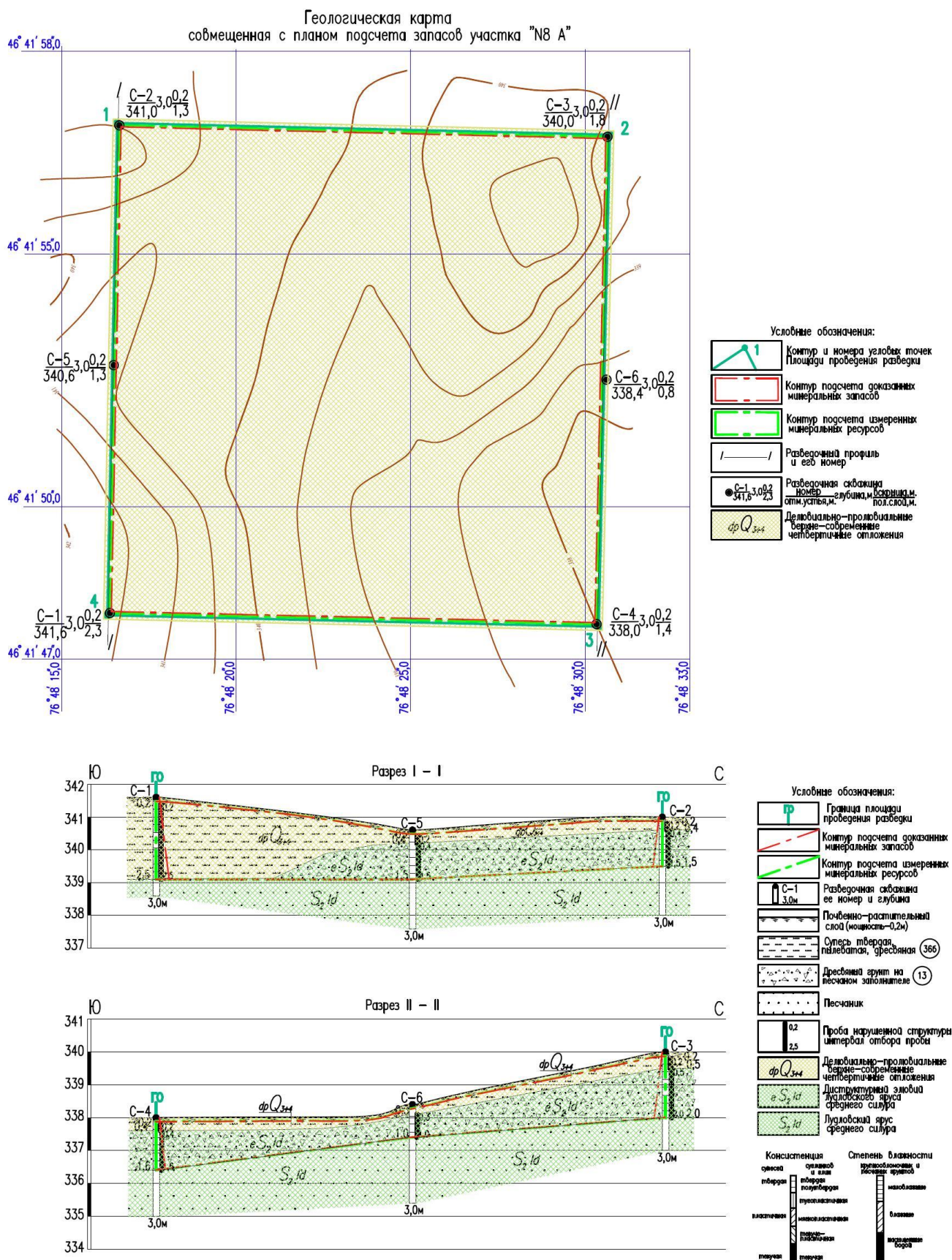
Рис. 2.7. Схема геологического строения участка №8А.
