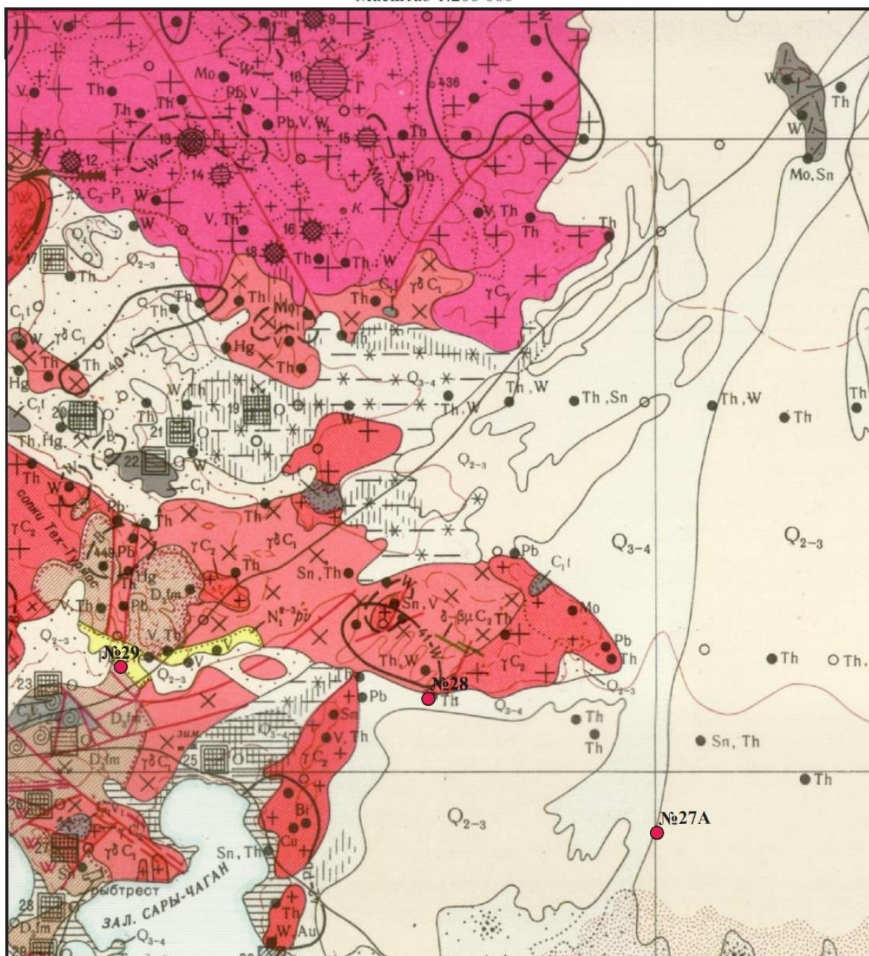
Рис.2.1 Геологическая карта расположения участков №29, №28, №27А. Масштаб 1:200 000
