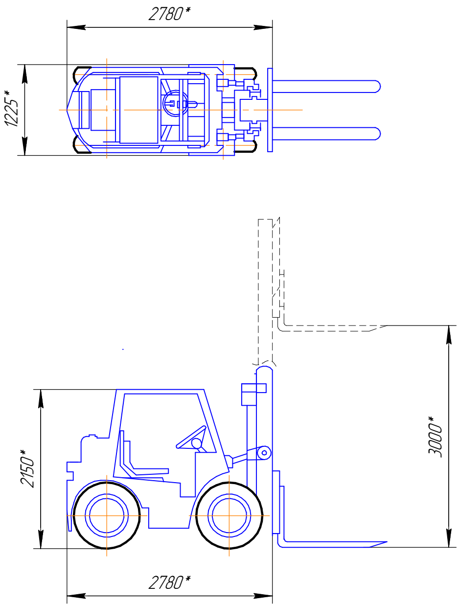
Вилочный погрузчик CPCD30-AG2 Масштаб 1:50
