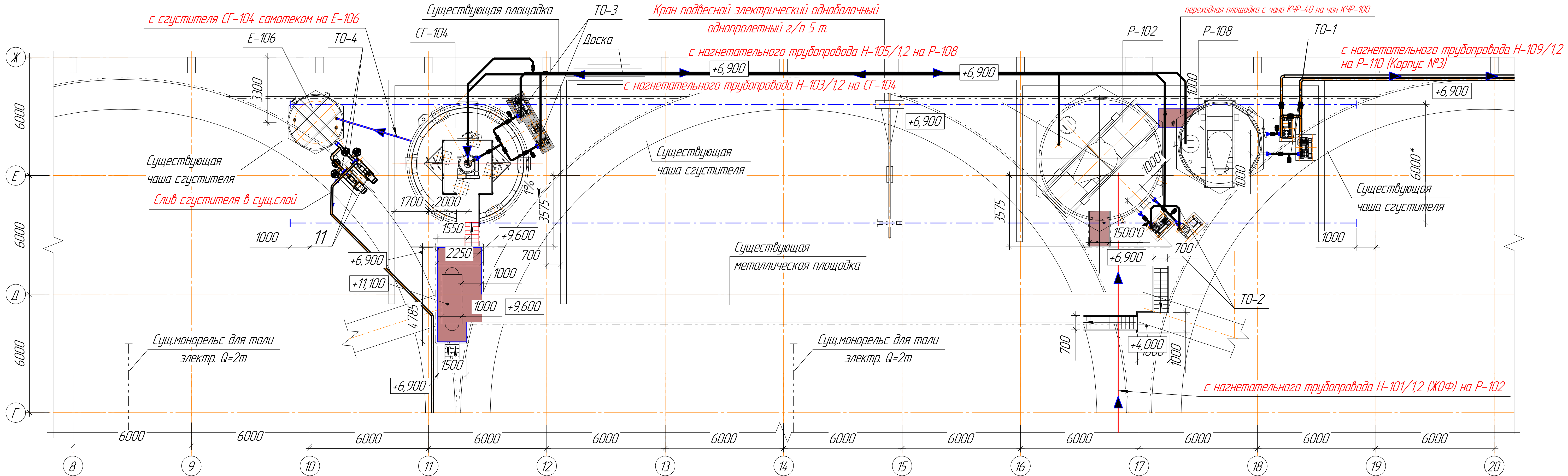
План установки технологических трубопроводов (1:100)
