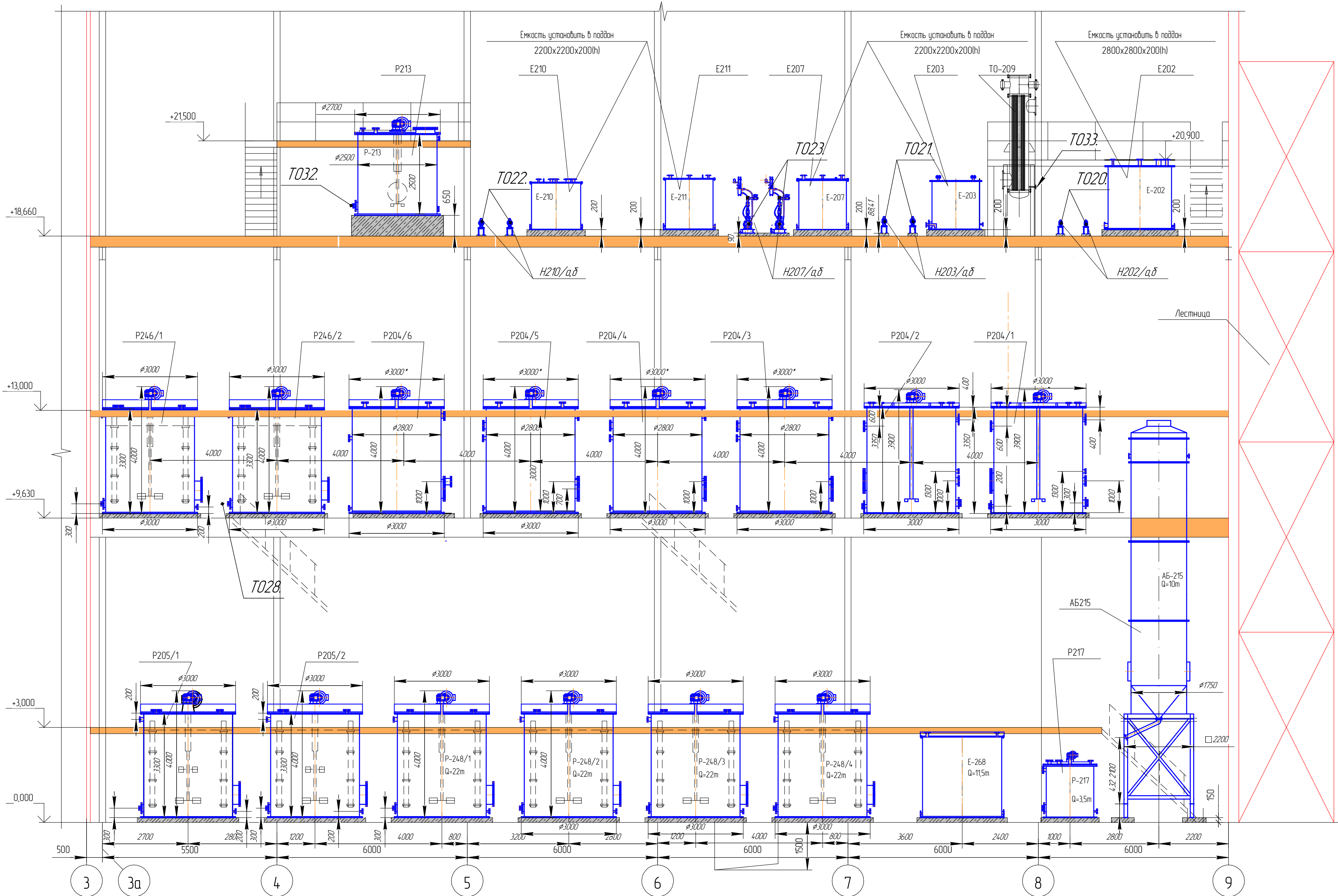
Б-Б (1:75)
