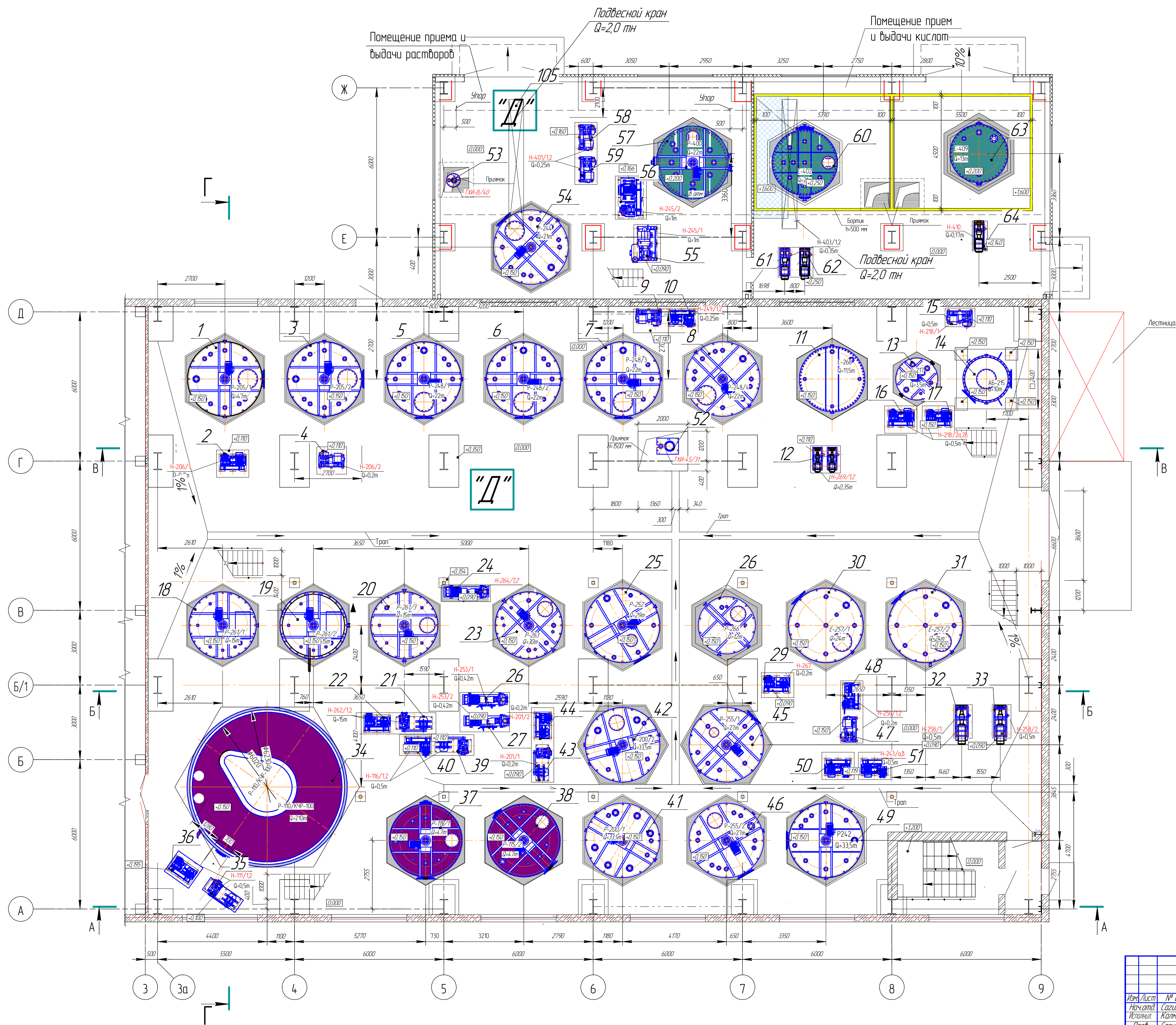
План (1:75)
