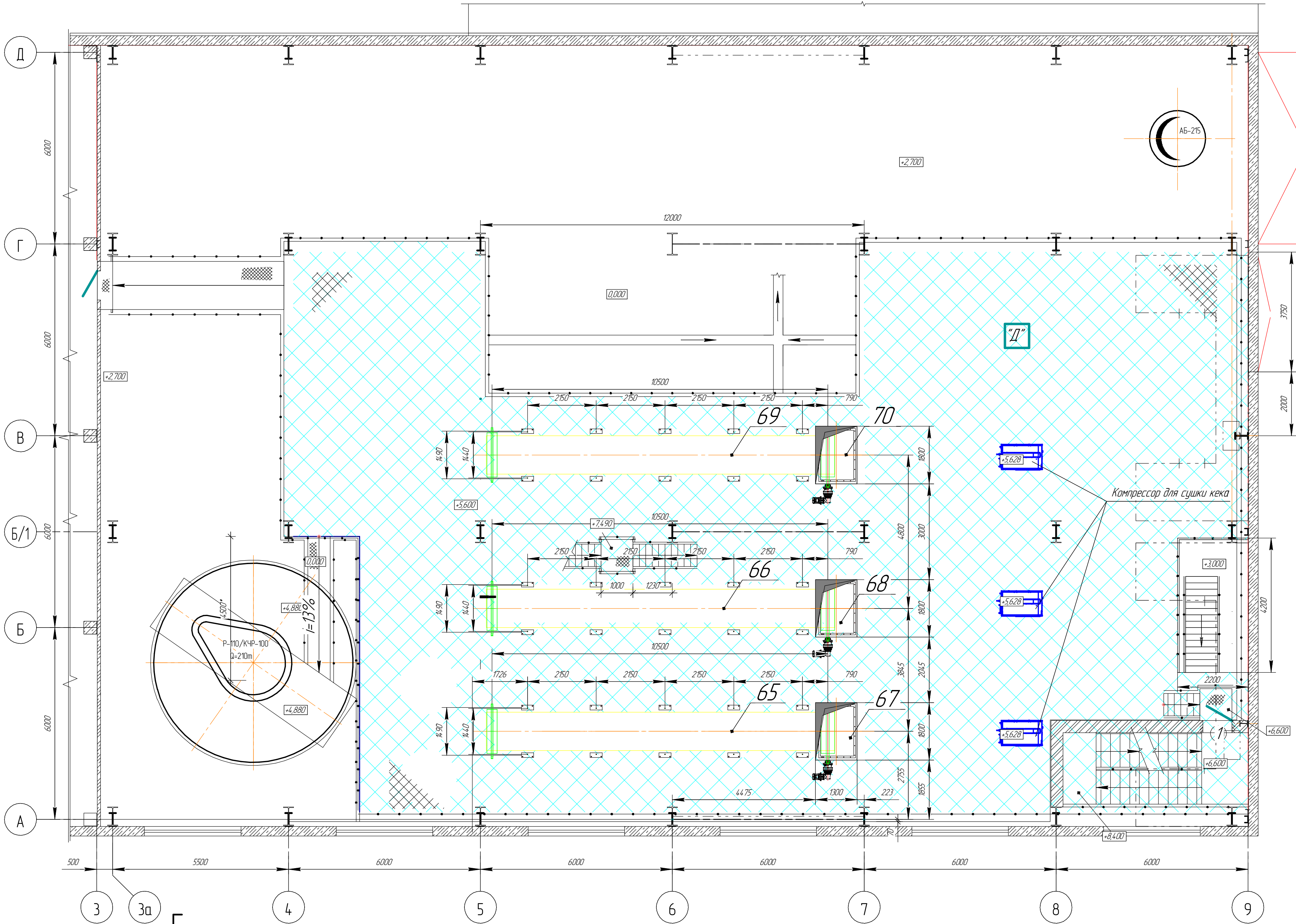
План на отм. +9,630
