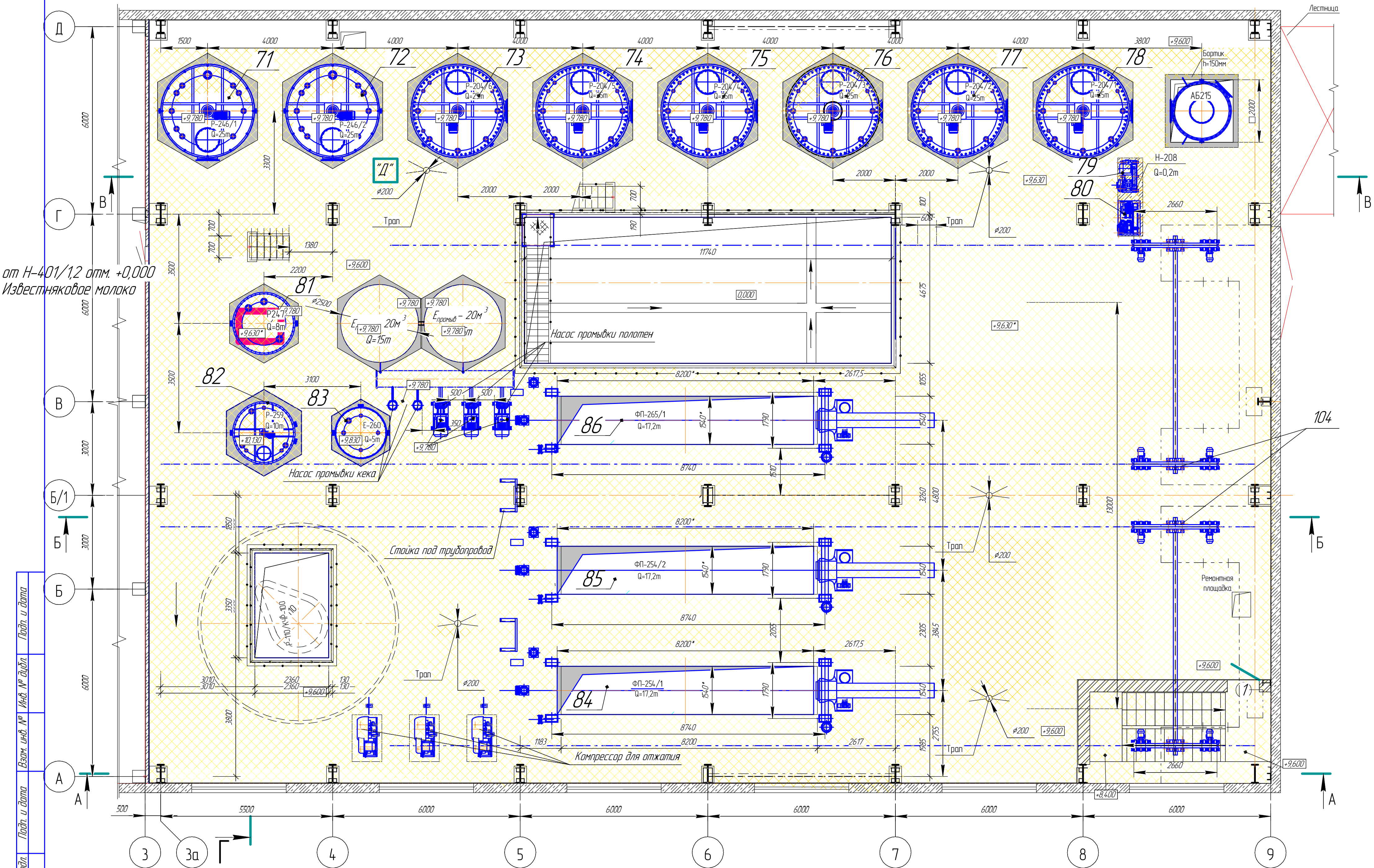
План на отм. +9,630
