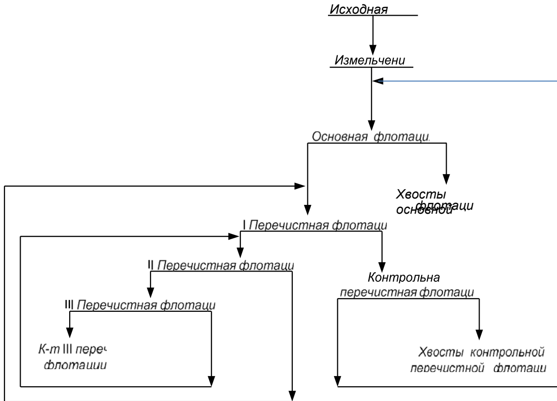
Рисунок 1.5.1 Технологическая схема для окисленной руды КР3 в масштабе промышленного предприятия согласно результатам испытаний для Рb
