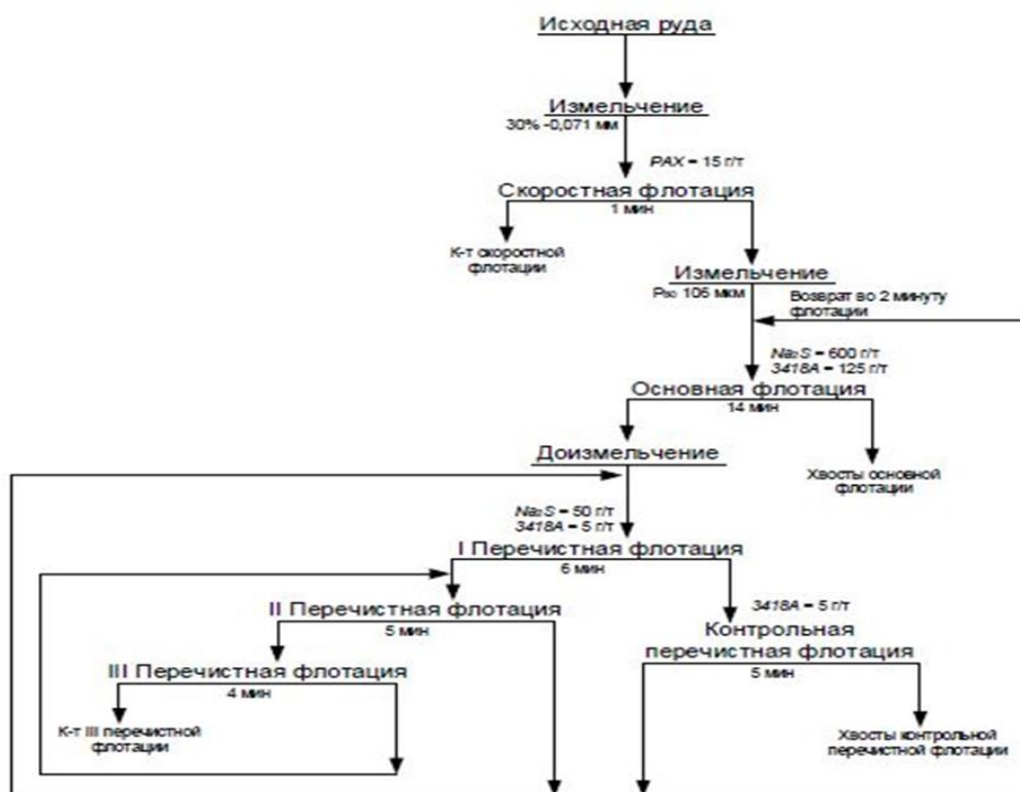
Схема обогащения сульфидной пробы руды месторождения Алайгыр по режиму Wardell Armstrong International
