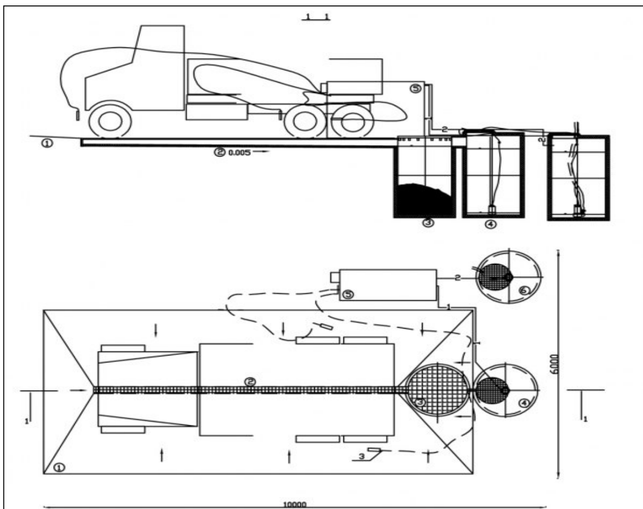
Схема применения установки оборотного водоснабжения мойки колёс грузовых автомобилей
