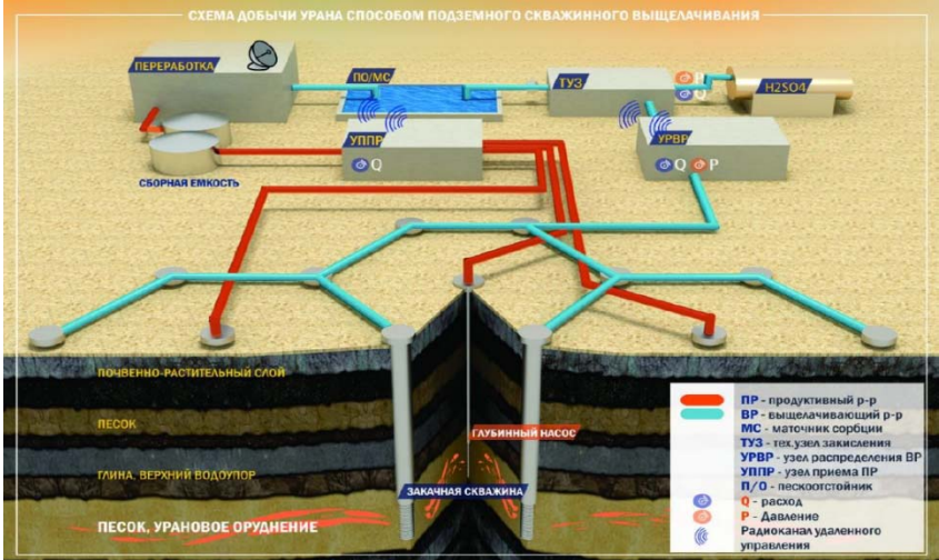
Рисунок 1.2 - Схема добычи и переработки урана методом ПСВ
