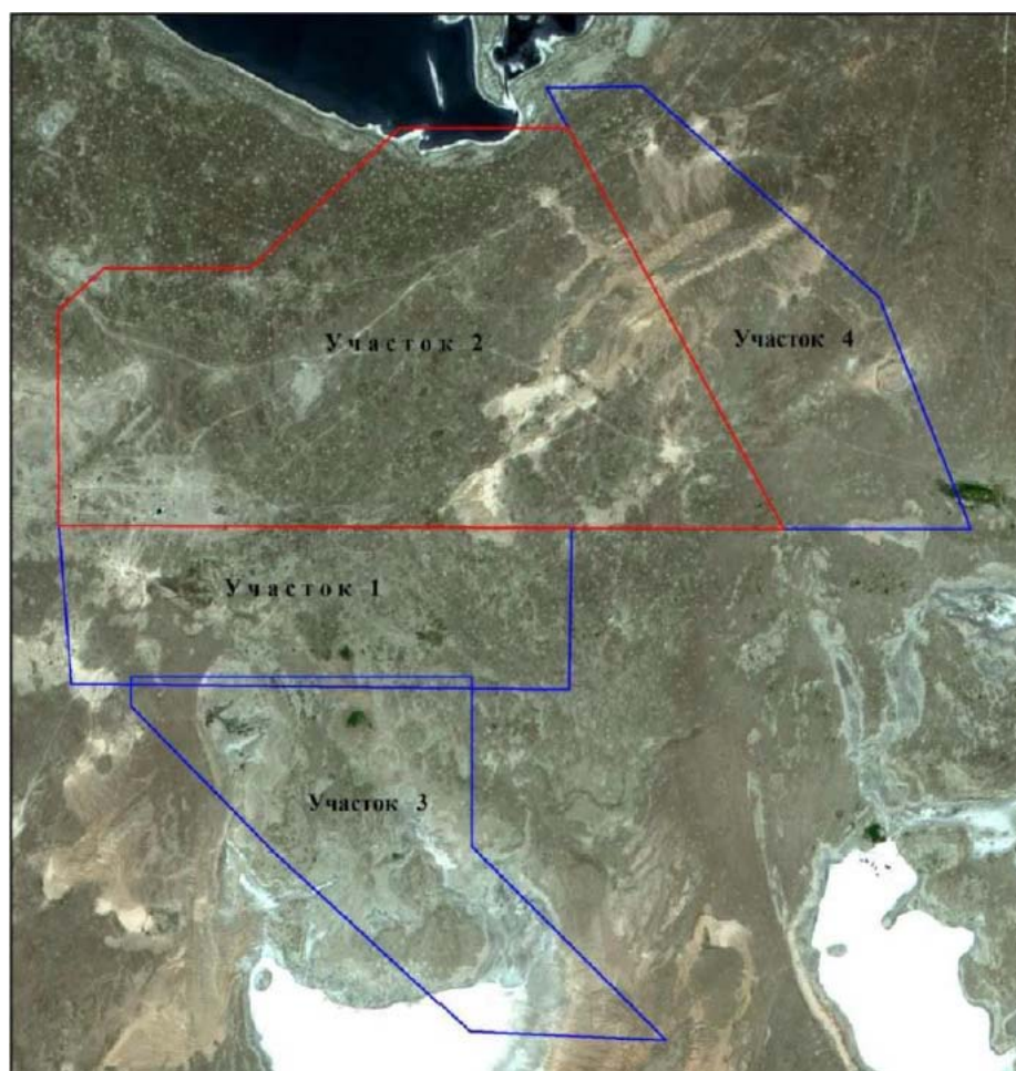
Рисунок 1.2 – Схема горного отвода участков №1,3,4 месторождения «Буденовское», обрабатываемых АО «СП «Акбастау»
