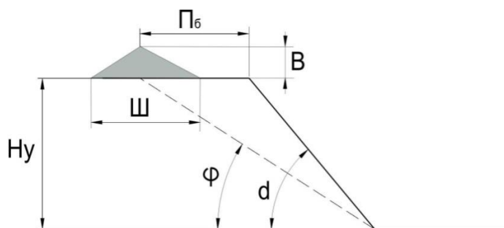
Рис.3.2.1 Схема уступа при отработке грунта
