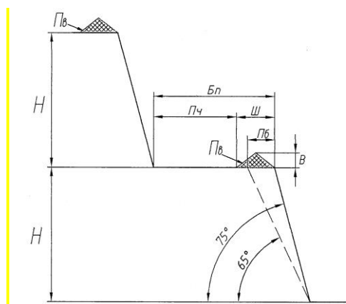
Рис.3.5.2 Схема уступа для участка строительного камня
