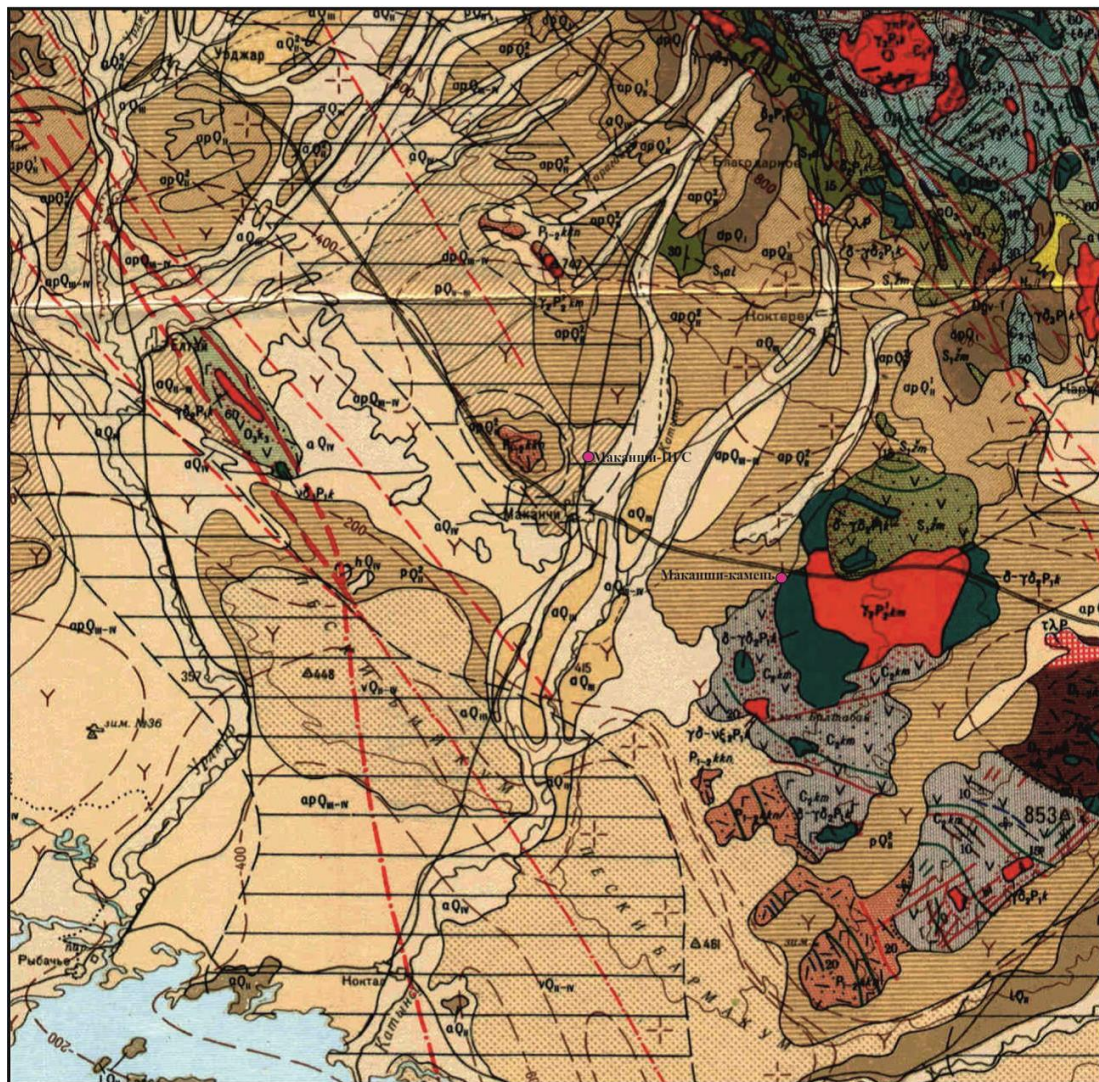
Рис.2.1. Геологическая карта района работ. Масштаб 1: 500 000
