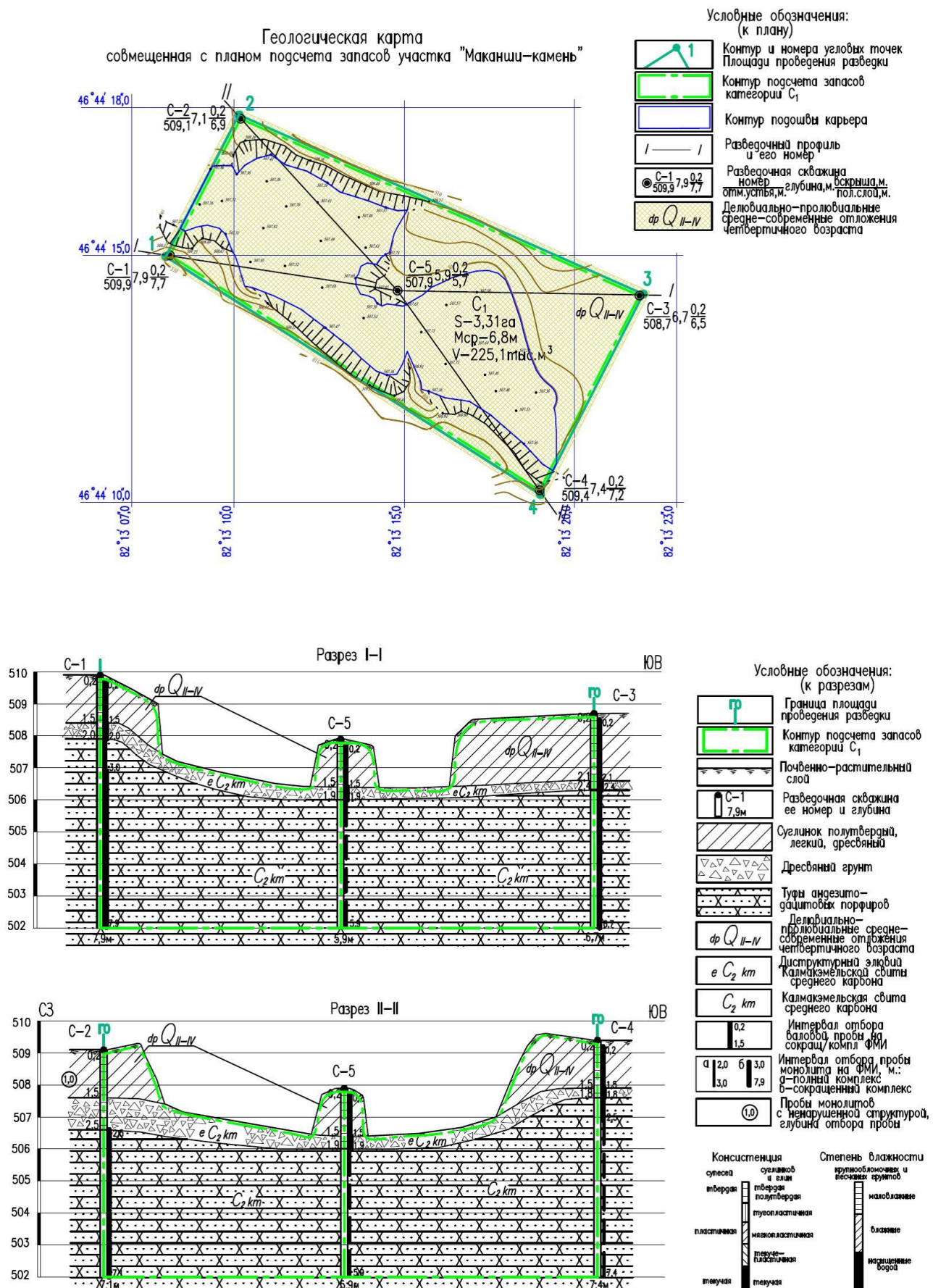
Рис.2.3 Схема геологического строения участка «Маканши-камень»
