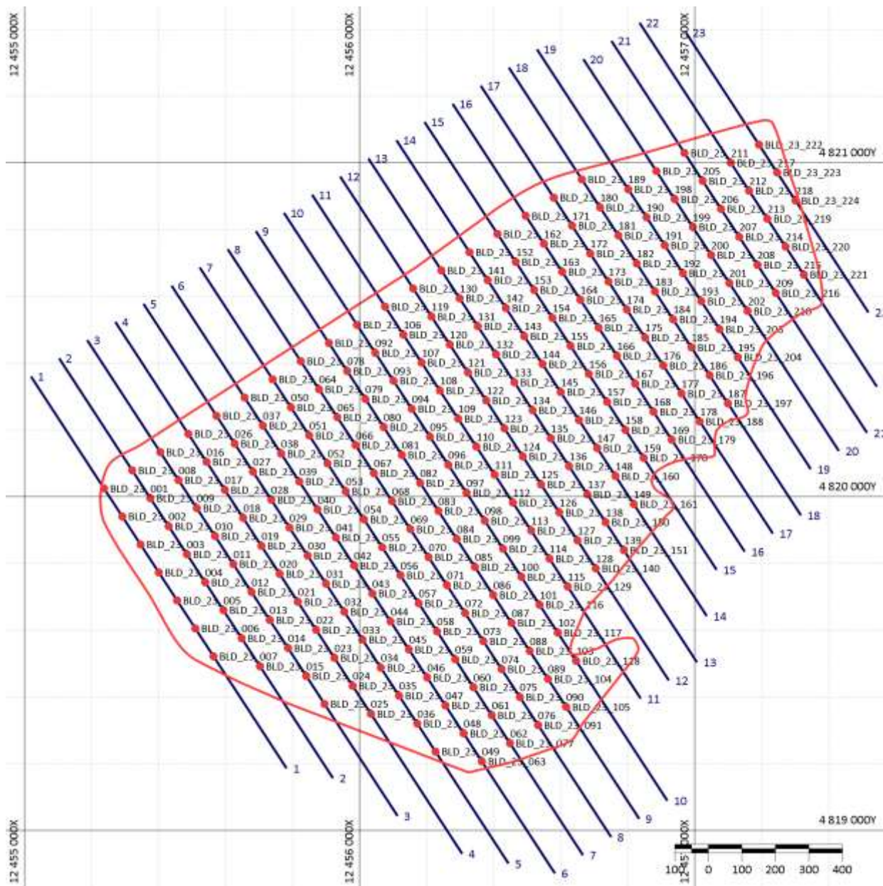
Рис. 6 - Схема расположения проектных скважин на Баялдырском хвостохранилище
