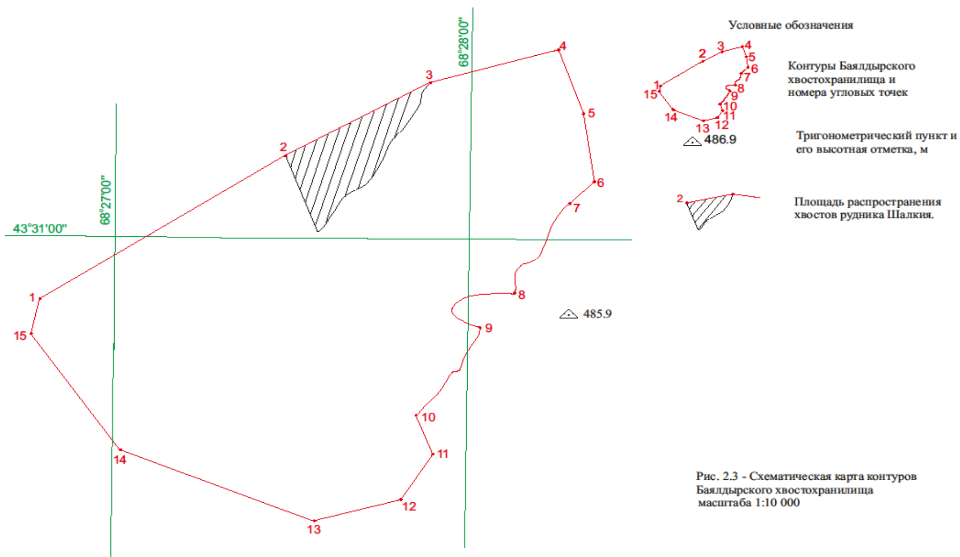
Рис. 2 – Схематическая карта контуров Баялдырского хвостохранилища масштаб 1:10 000
