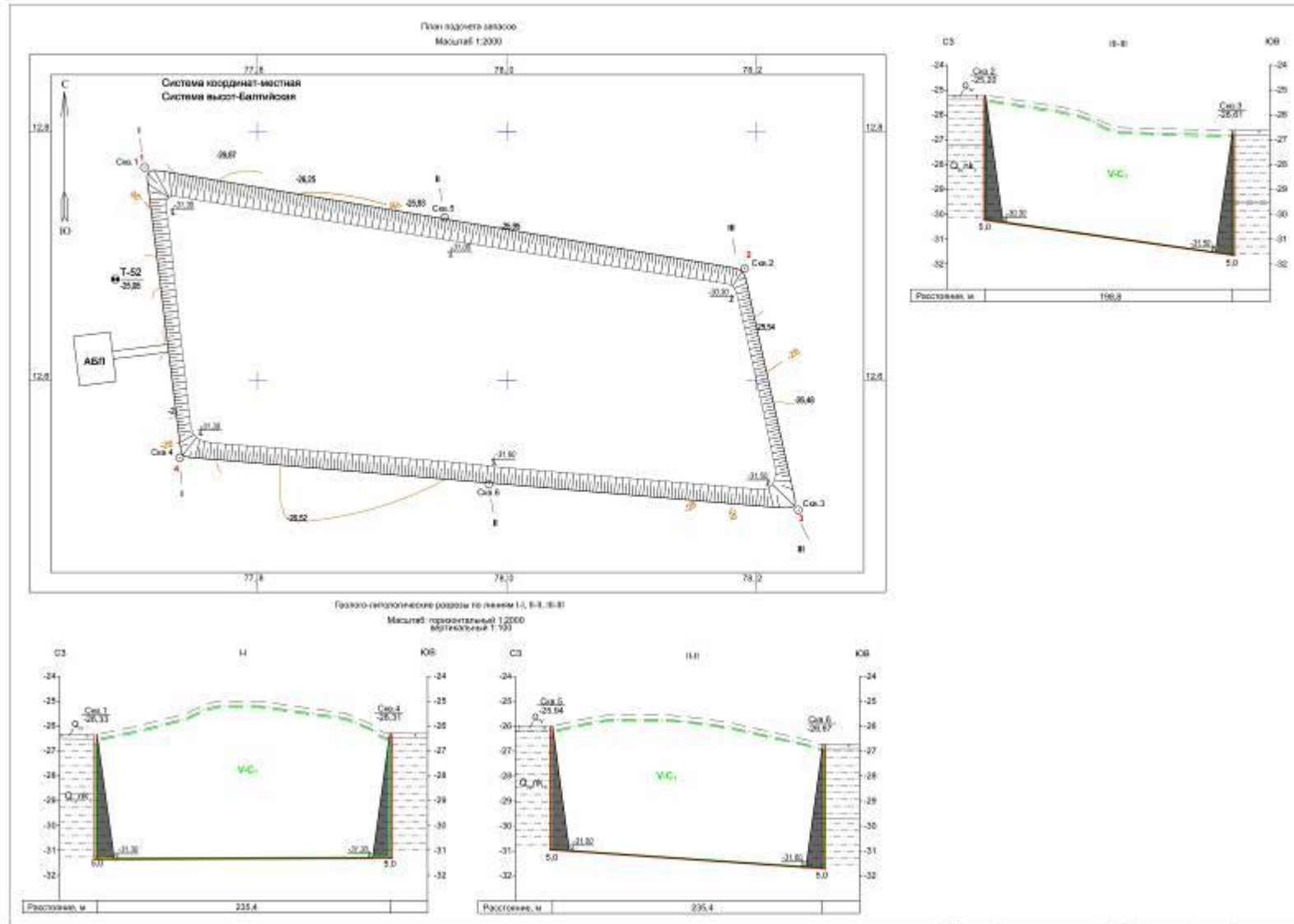
Рис.7. План карьера ГР №5 на конец погашения запасов
