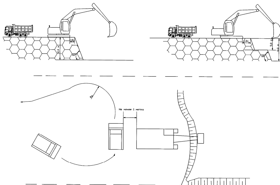
Рис.3. Технологическая схема отработки уступа с верхней погрузкой
