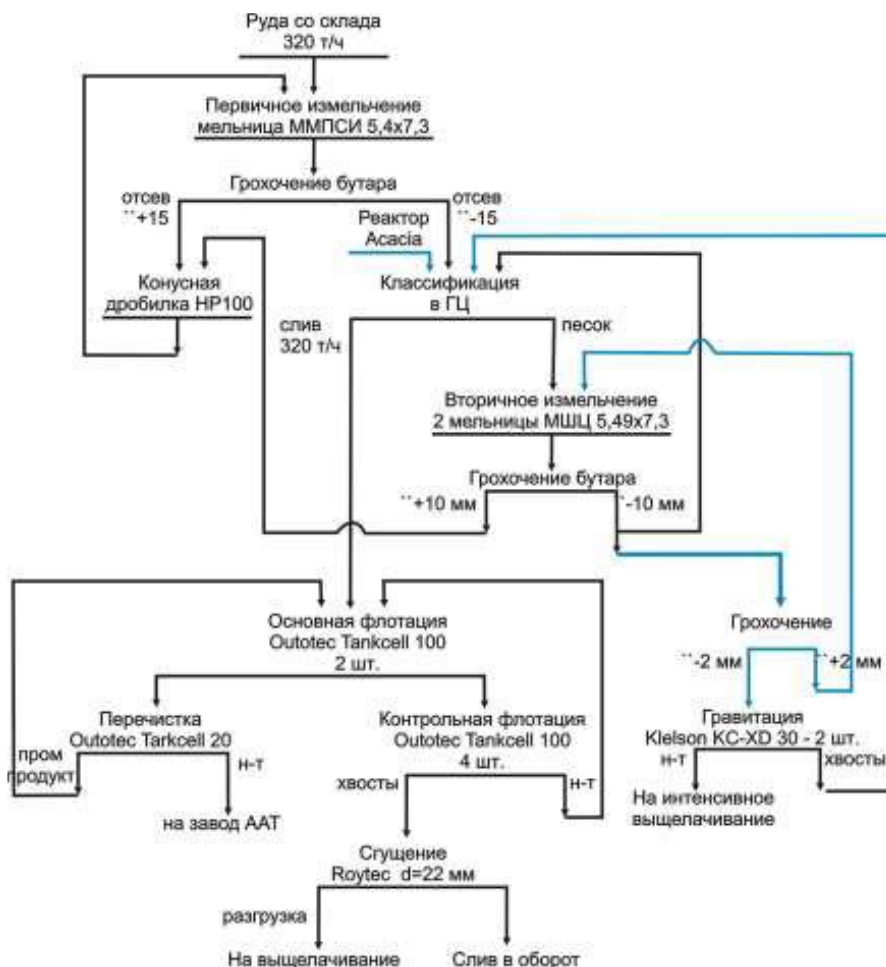
Рисунок 0.1 -Технологическая схема измельчения, классификации, гравитации и флотации
