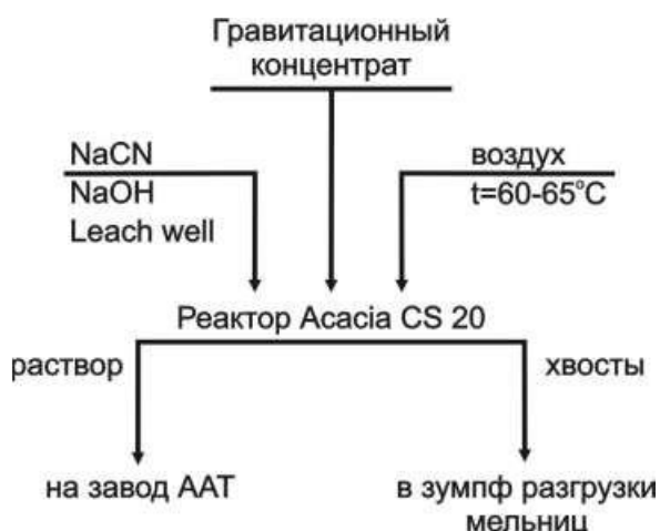
Рисунок 0.2 - Технологическая схема выщелачивания золота из гравитационного
