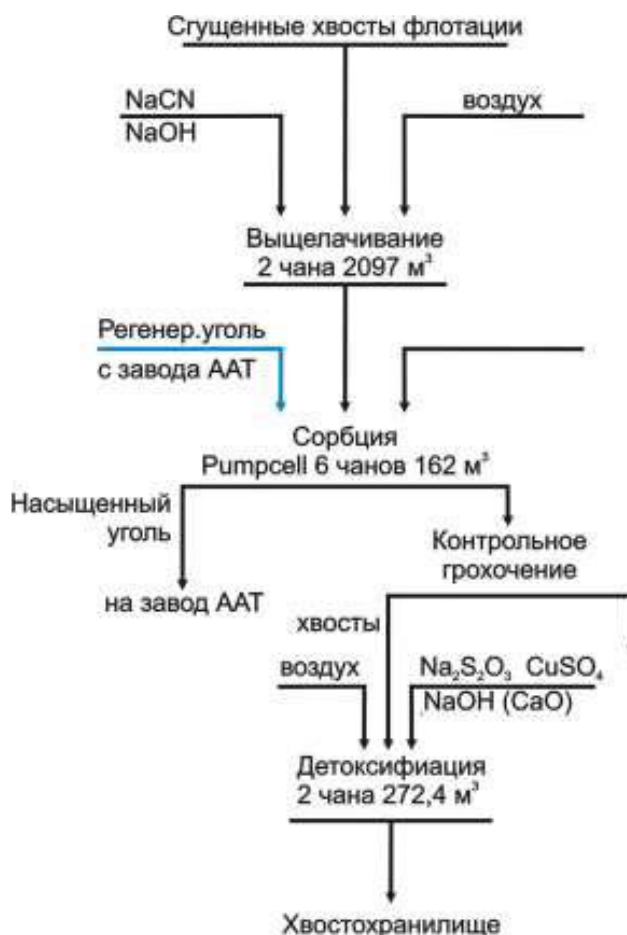
Рисунок 0.3 - Технологическая схема выщелачивания золота из гравитационного концентрата
