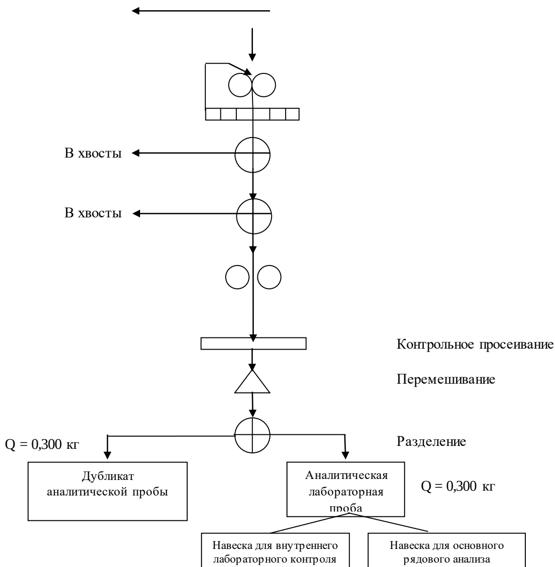
Рис. 4.2 Схема обработки керновых проб
