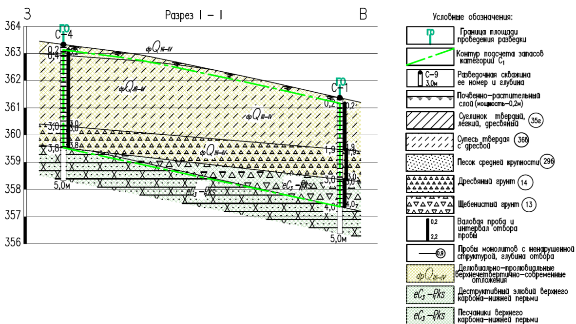
Рис. 2.6. Схема геологического строения участка «№4 А жд, ПК1191»
