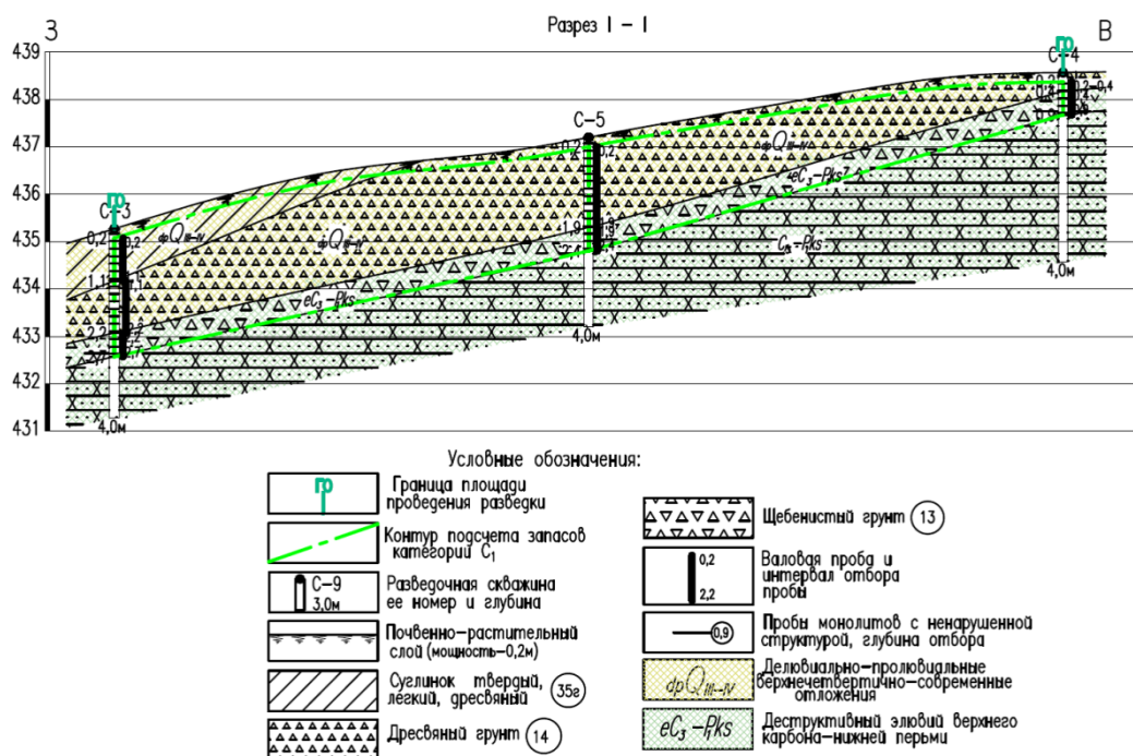
Рис. 2.5 Схема геологического строения участка «№4 В жд, ПК1165».
