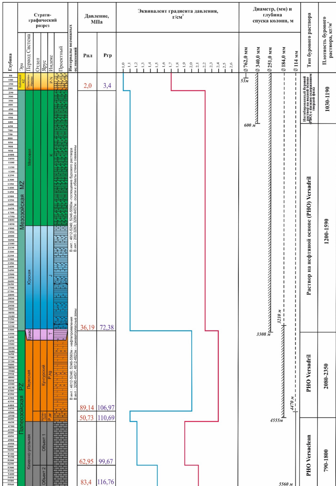
Рисунок 3.1. График совмещенных давлений по колоннам скважины Т-6549
