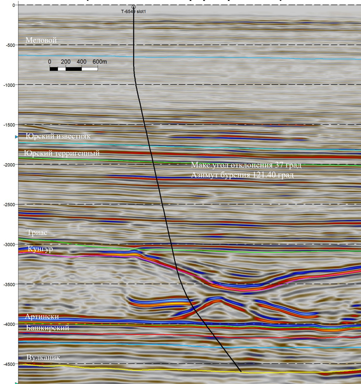
Рисунок 1.4. Сейсмический разрез через скважину Т-6549
