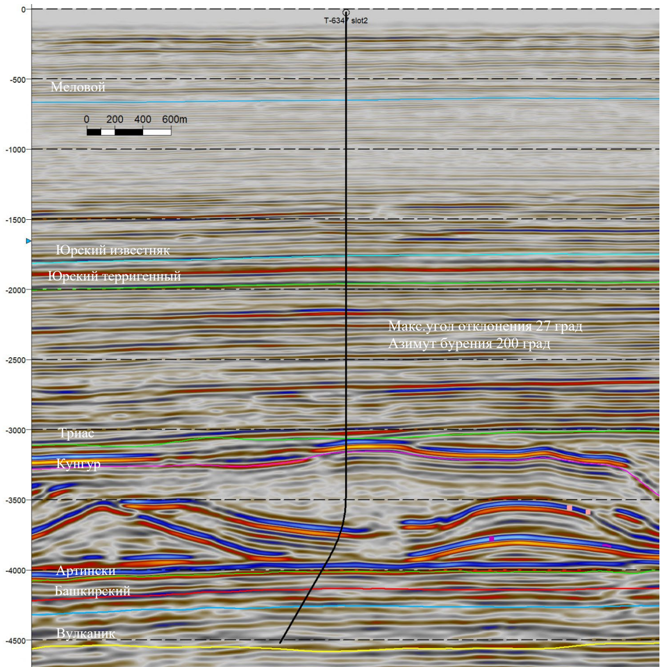
Рисунок 1.4. Сейсмический разрез через скважину Т-6347
