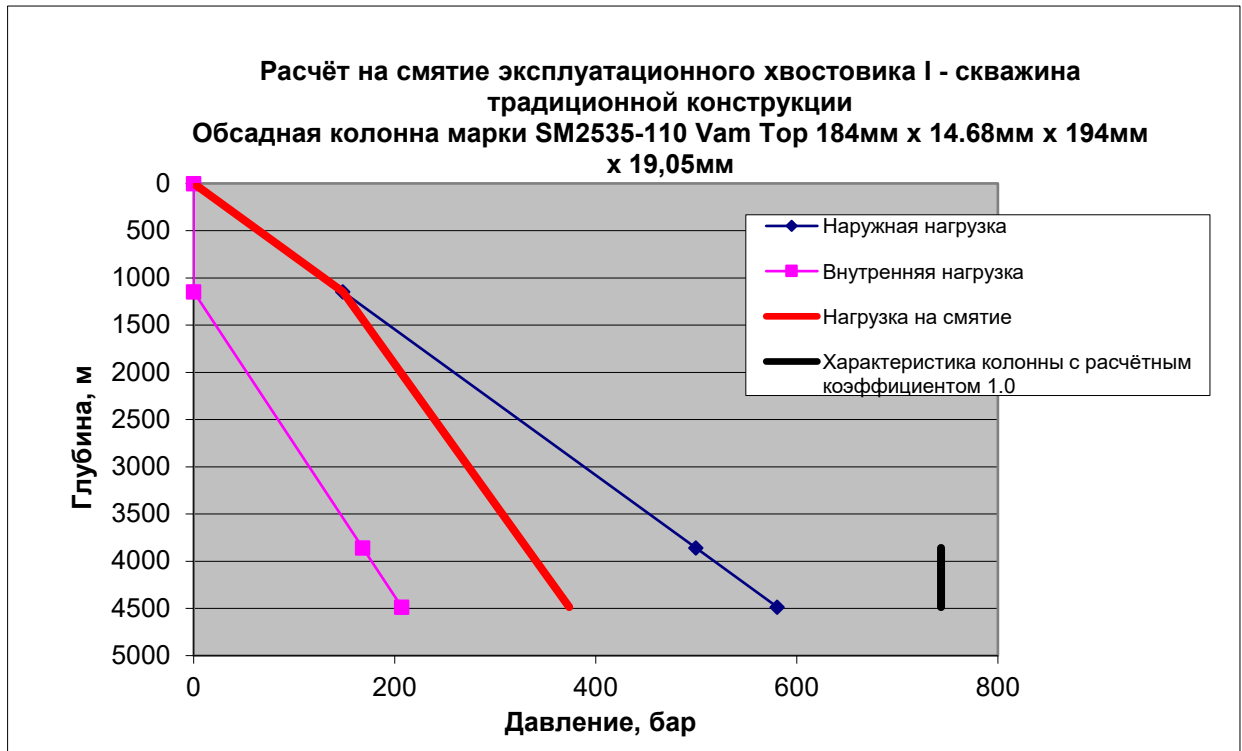
Диаграмма 8.3. Скв. Т-4662. Эксплуатационный хвостовик I
