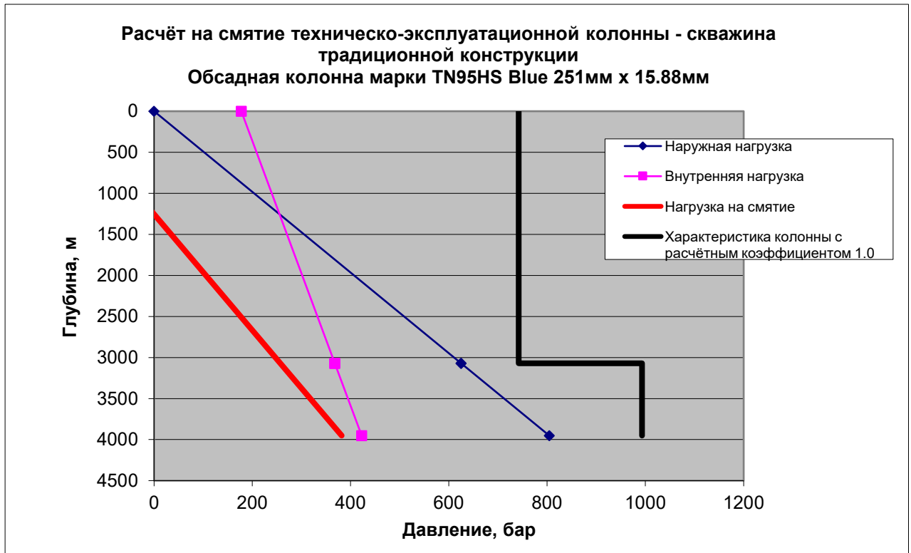
Диаграмма 8.2. Скв. Т-4662. Техническо-эксплуатационная колонна
