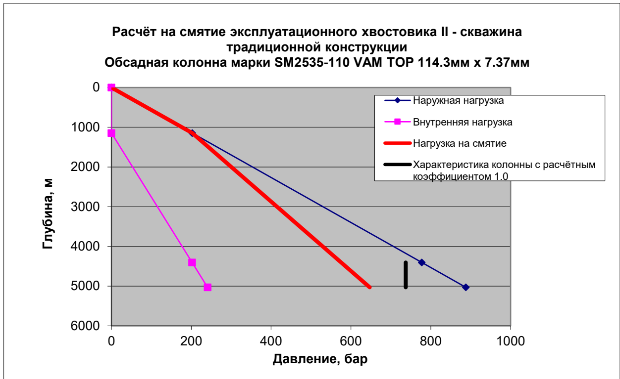
Диаграмма 8.4. Скв. Т-4662. Эксплуатационный хвостовик II
