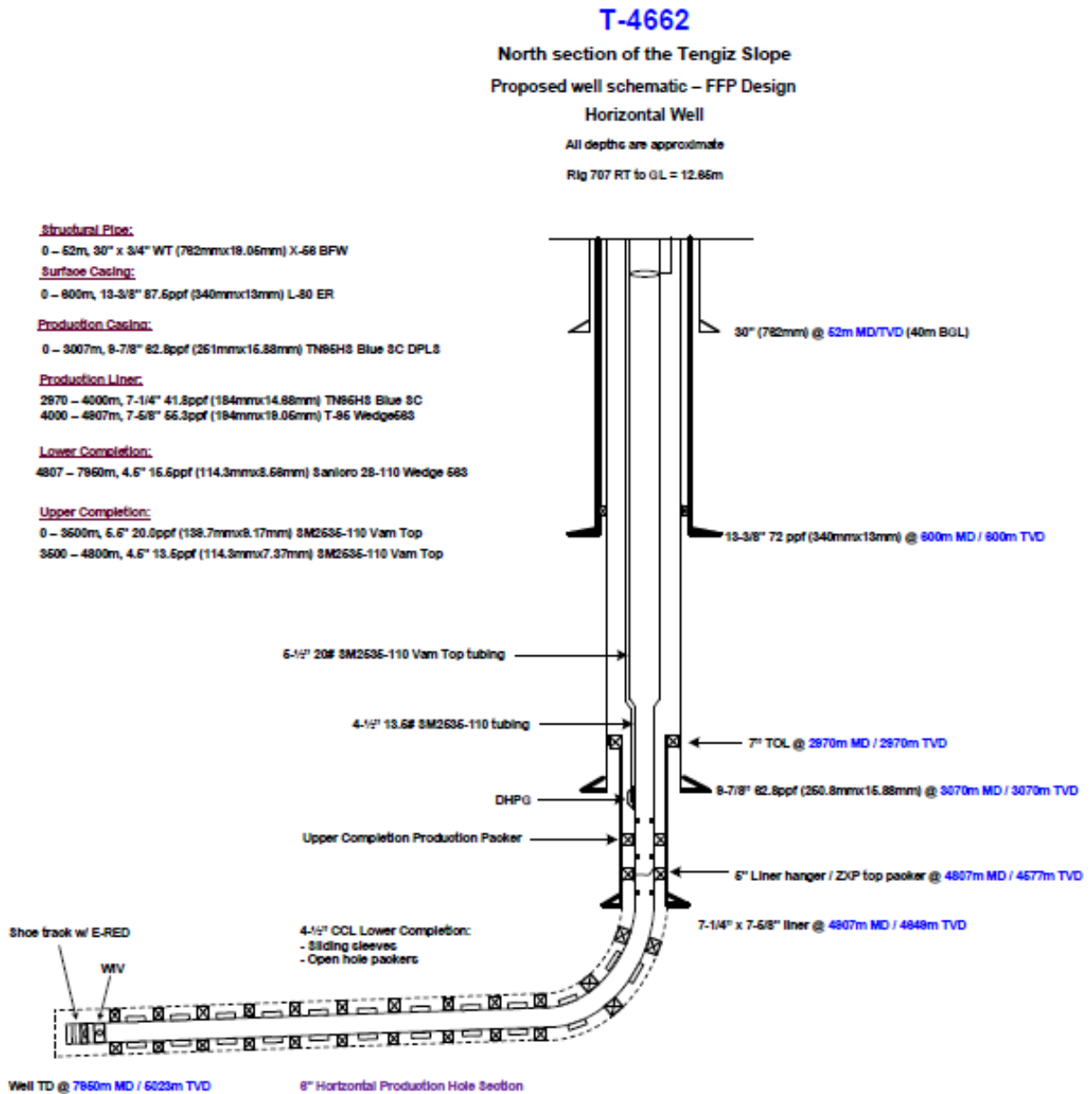
Рисунок 8.1. Скв. Т-4662 Схема ствола скважины
