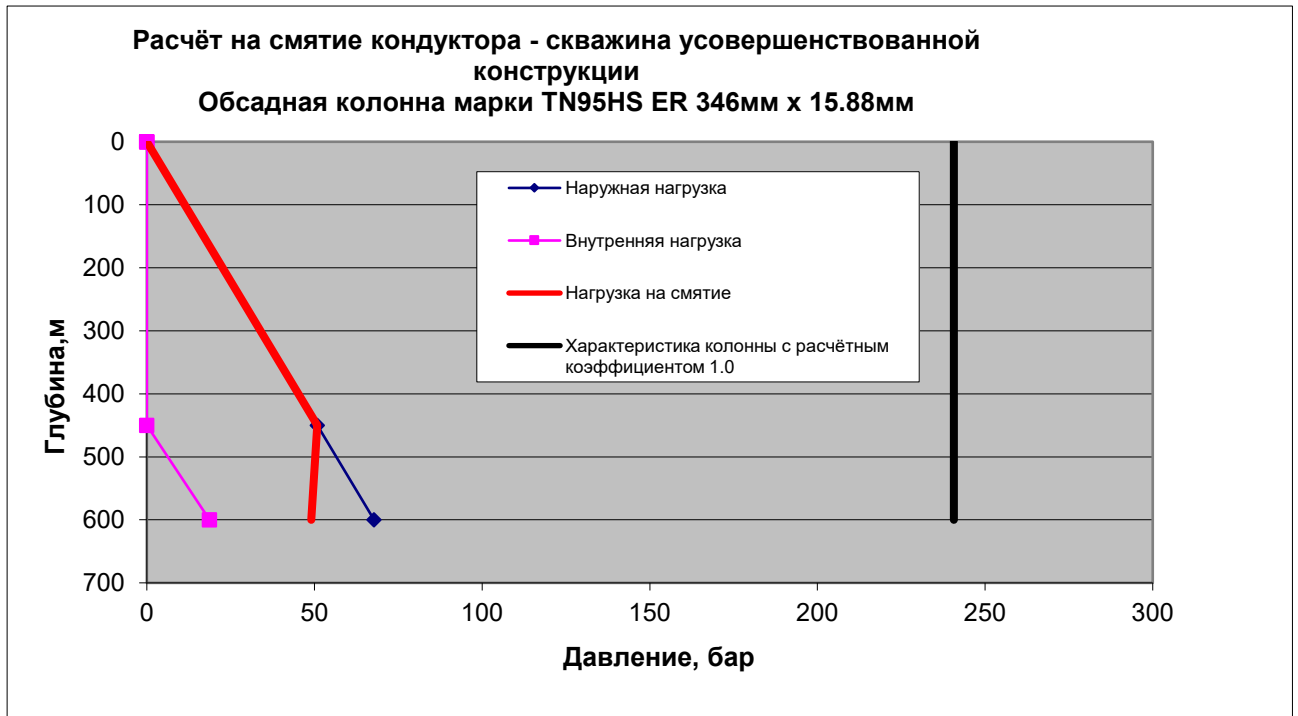
Диаграмма 8.1. Скв. Т-4662. Кондуктор
