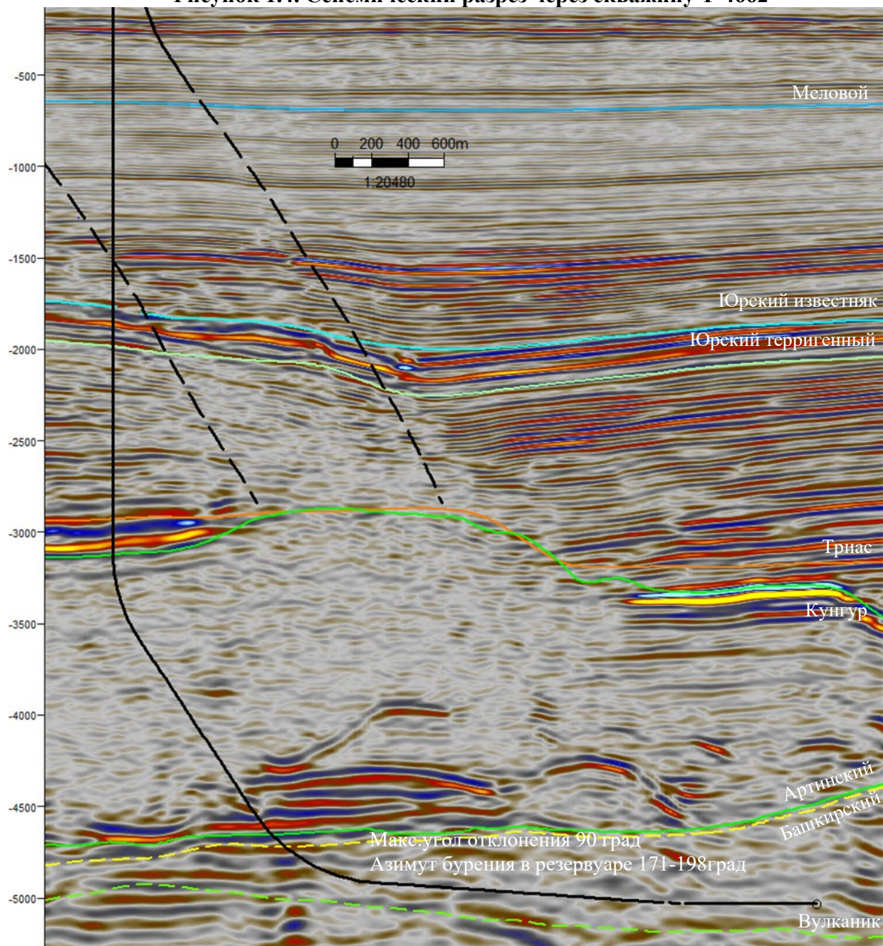
Рисунок 1.4. Сейсмический разрез через скважину Т-4662
