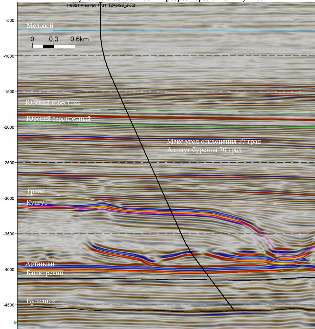
Рисунок 1.4. Сейсмический разрез через скважину Т-6351
