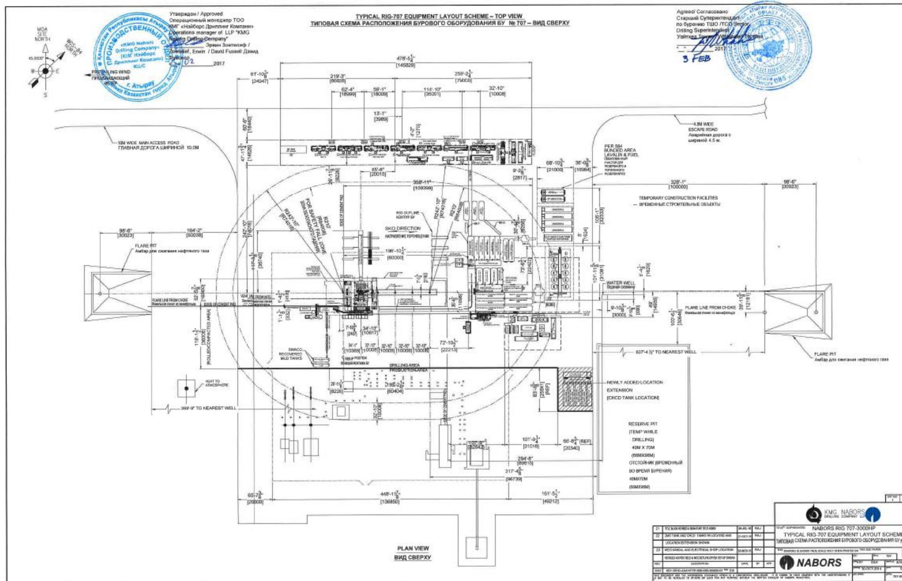
Приложение 14. Типовая схема расположения бурового оборудования на БУ №707 (1 из 3)
