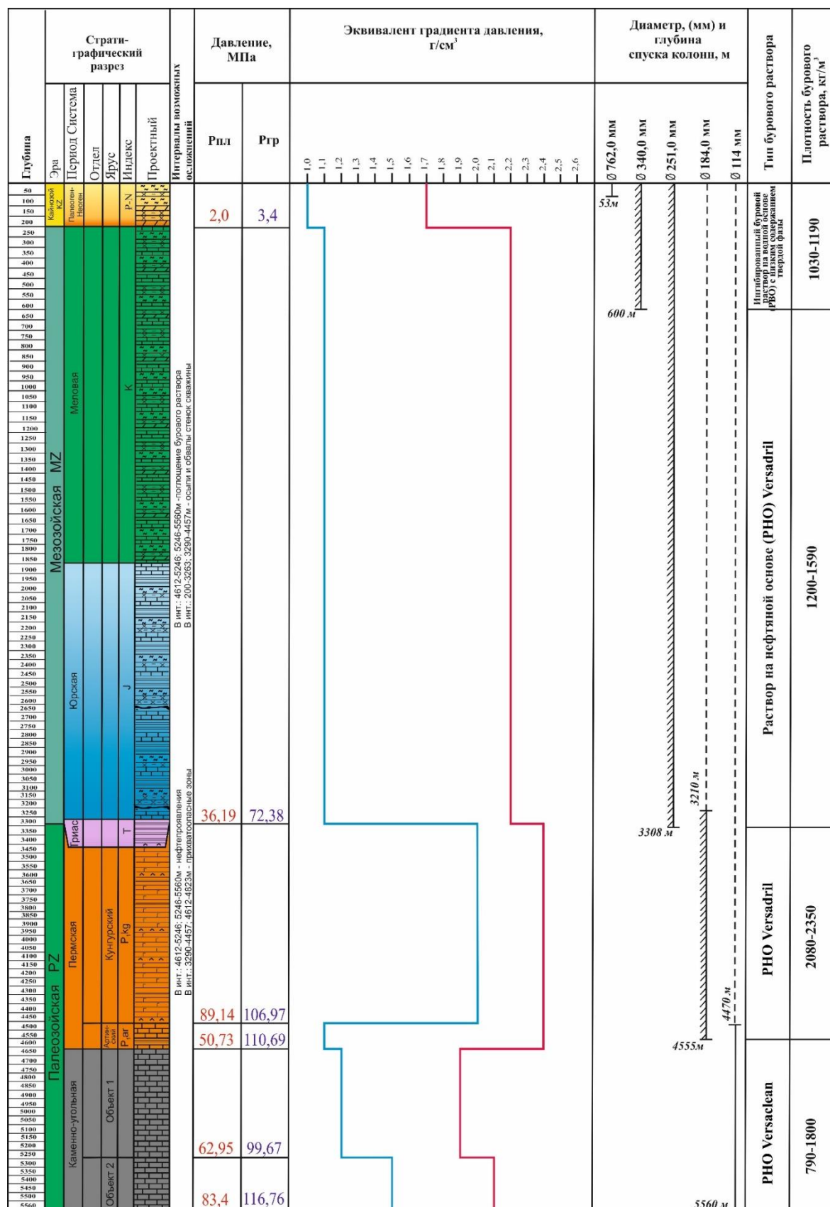
Рисунок 3.1. График совмещенных давлений по колоннам скважины Т-6351
