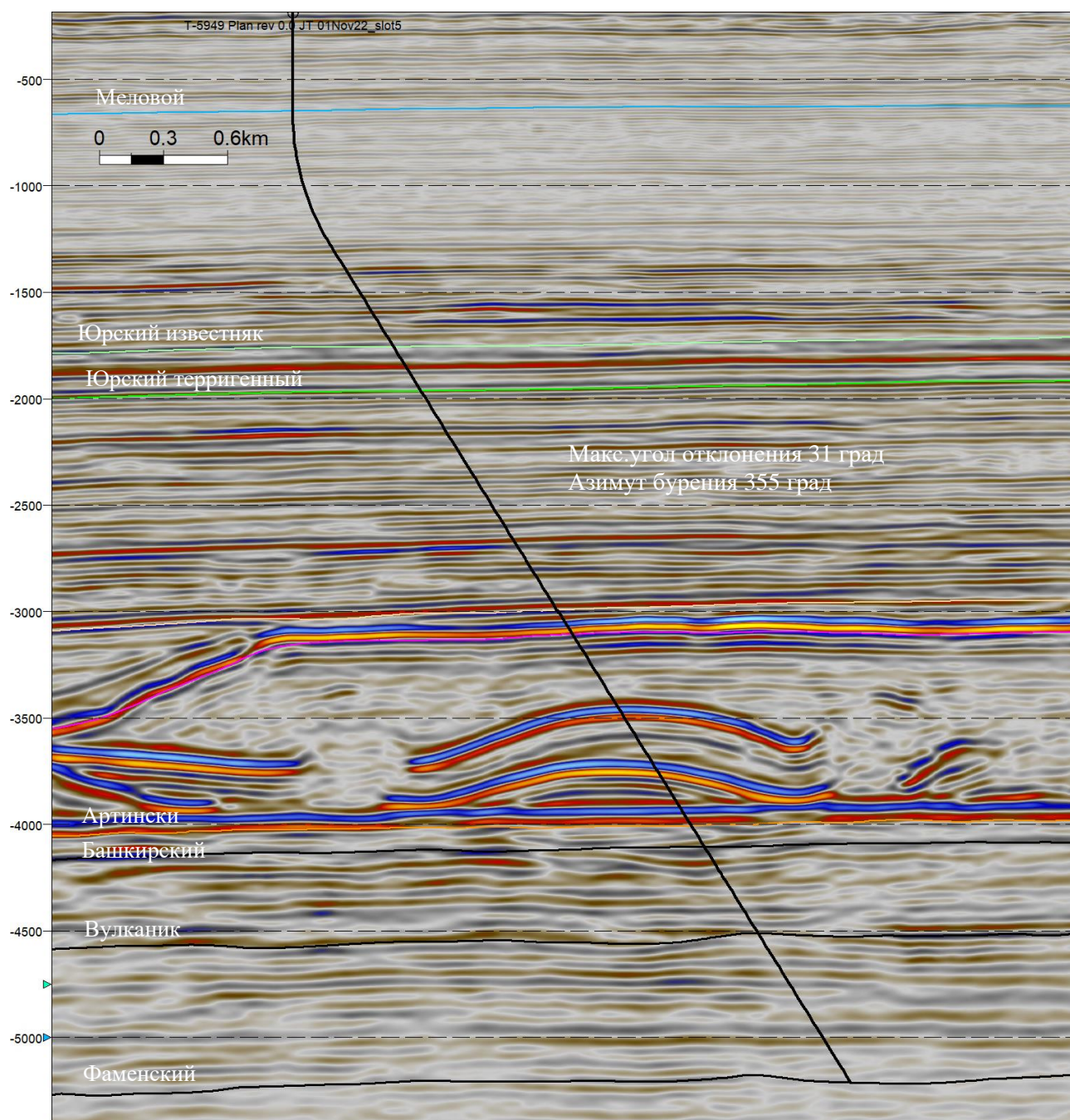
Рисунок 1.4. Сейсмический разрез через скважину Т-5949
