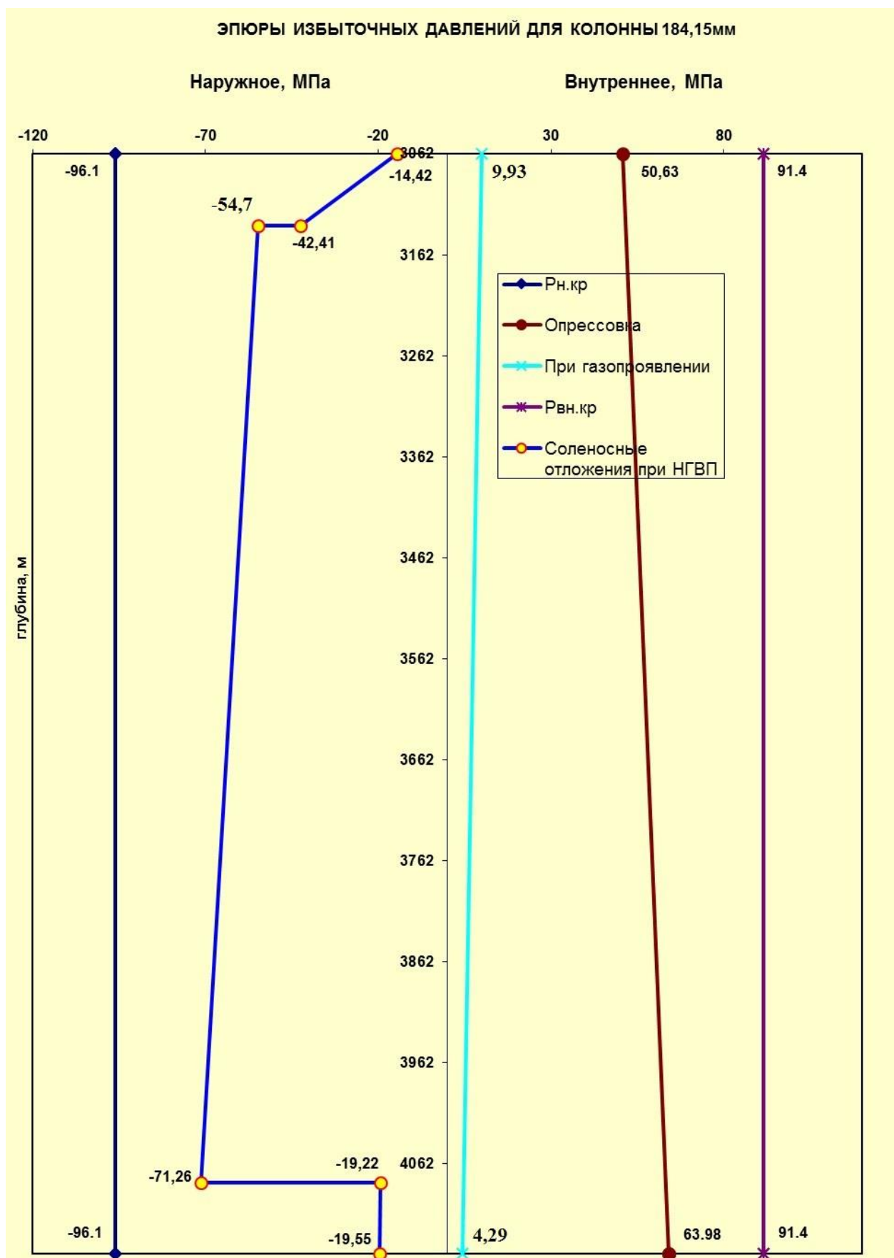
Рисунок 1.9 Эпюра избыточных давлений для колоонны Ø184,15мм
