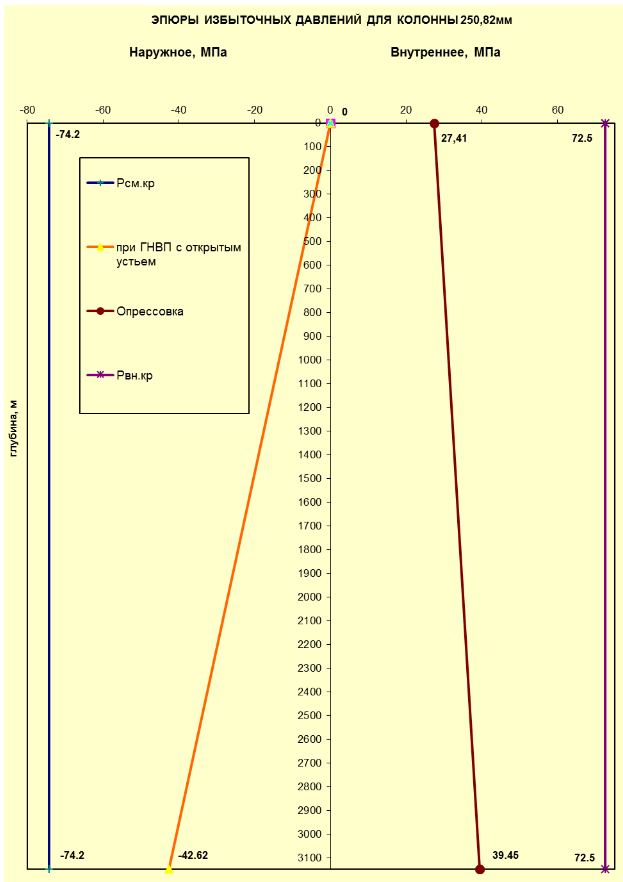
Рисунок 1.8 Эпюра избыточных давлений для колоонны Ø250,8мм
