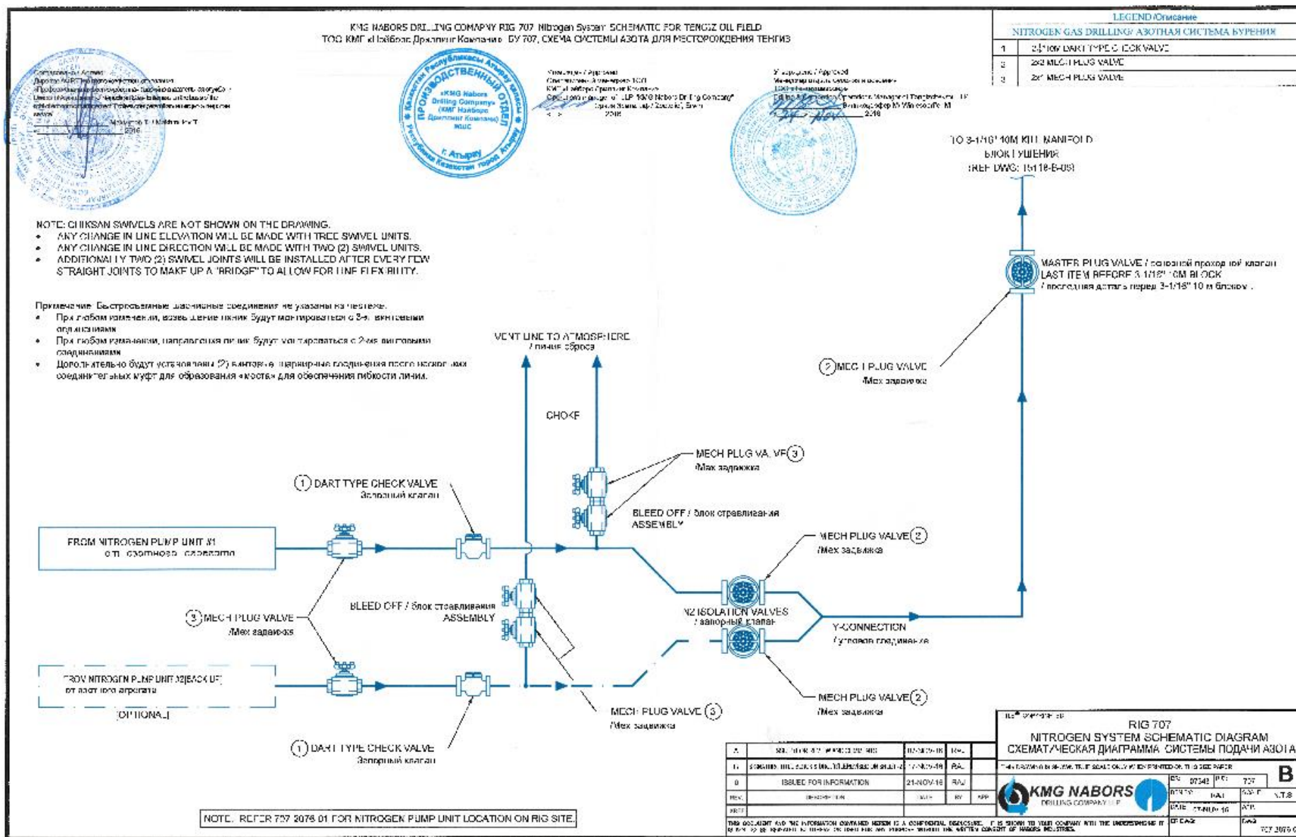
Приложение 13. Бурение с применением азота. Типовая схематическая диаграмма системы подачи азота (1 из 2)
