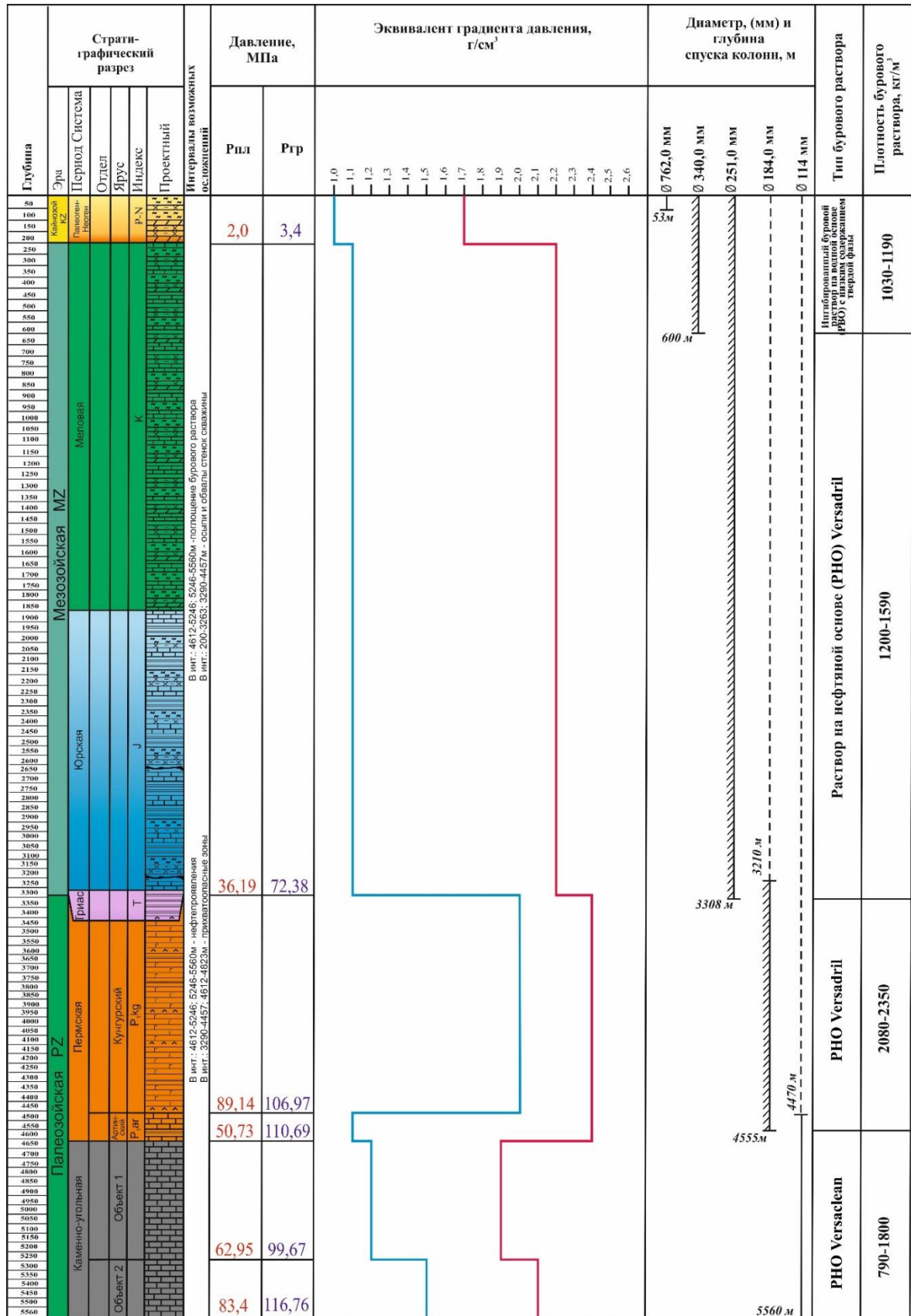
Рисунок 3.1. График совмещенных давлений по колоннам скважины Т-5341
