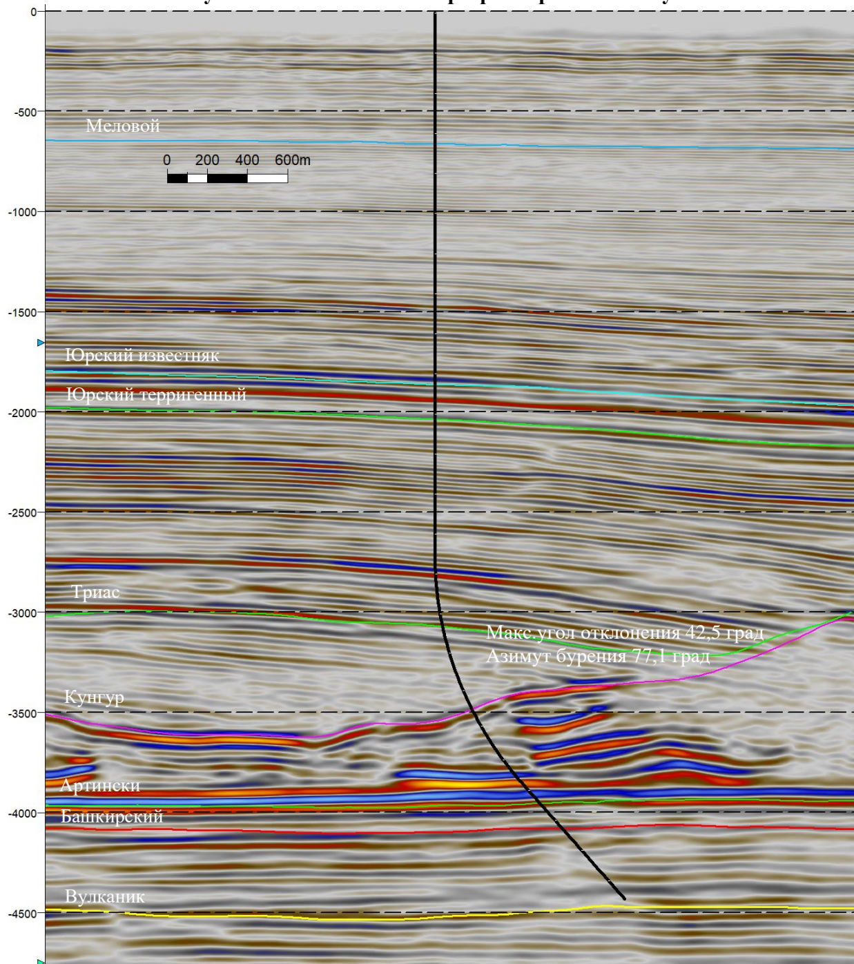
Рисунок 1.4. Сейсмический разрез через скважину Т-5147
