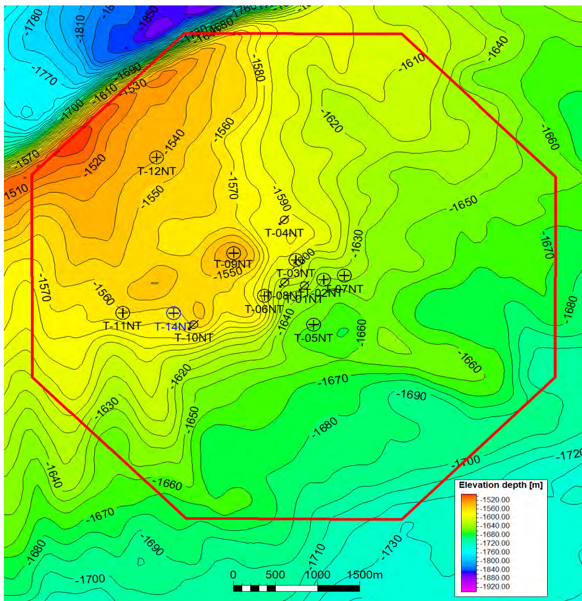
Рисунок 1.2 - Карта месторождения Тенгиз с указанием участка закачки сточных вод, показывающая местоположение предлагаемой скважины Т-14NT, а также местоположение существующих водопоглощающих скважин
