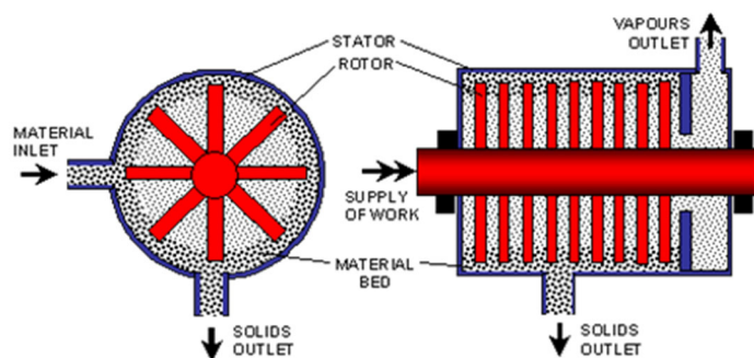
Рисунок 2.5 Принципиальная схема работы установки ТСС
