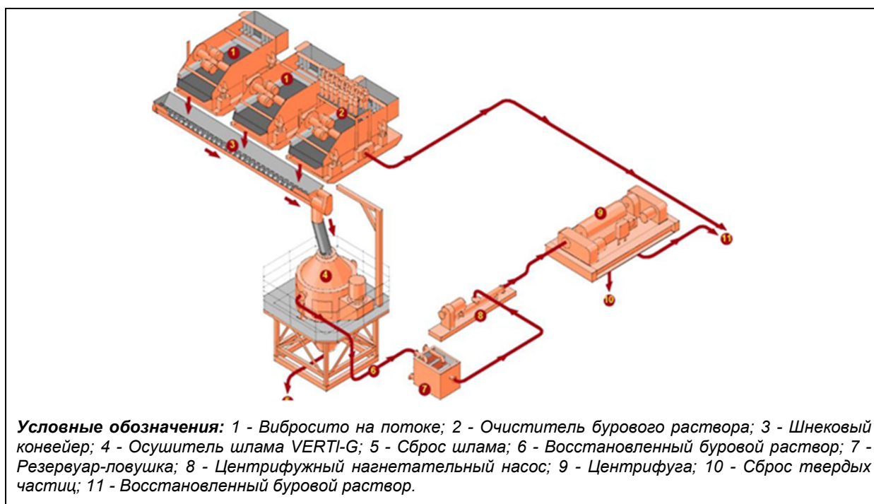
Рисунок 2.6 Принципиальная схема работы установки VERTI-G
