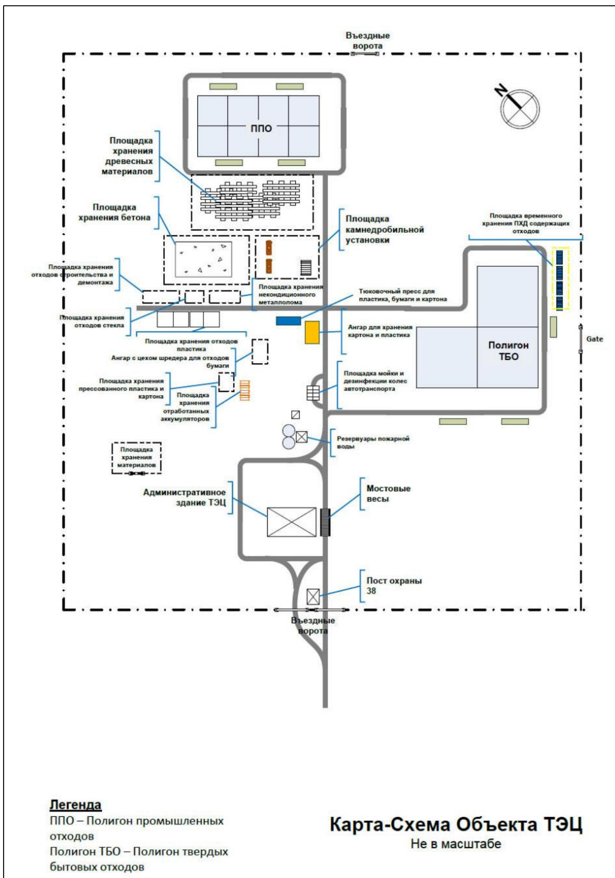
Рисунок 1.12 Схема расположения объектов ТЭЦ
