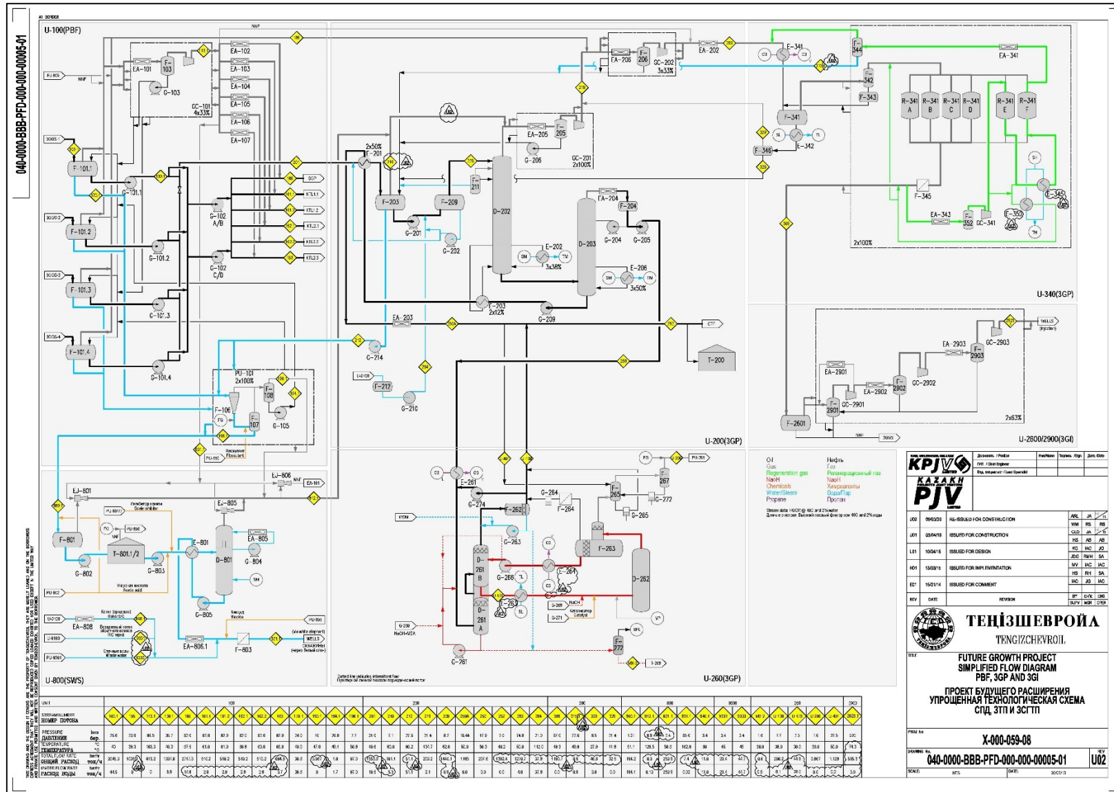
Рисунок 1.9 Упрощенная технологическая схема ПБР
