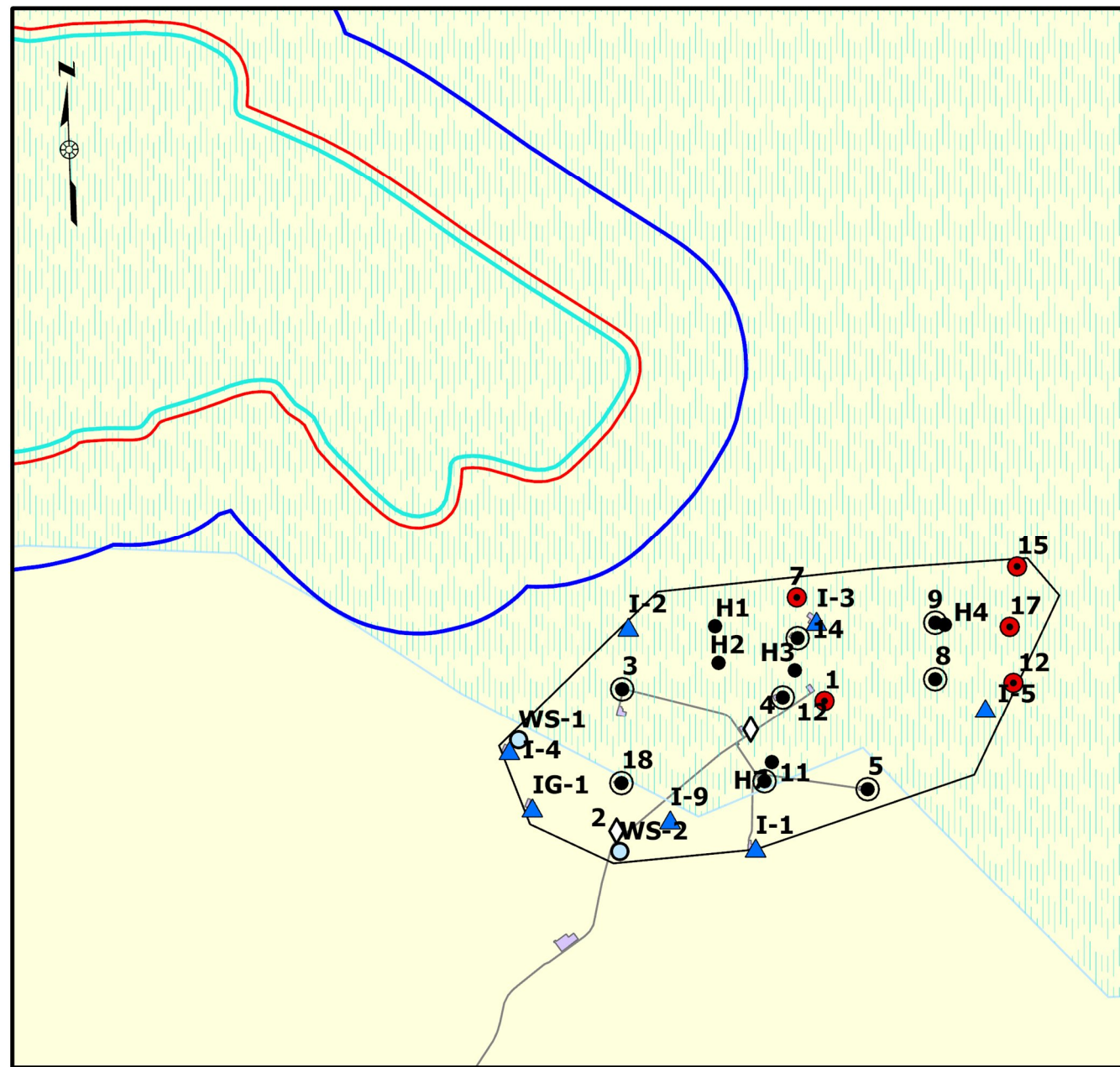
Рисунок 2 - Схема расположения пробуренных скважин на месторождении Комсомольское
