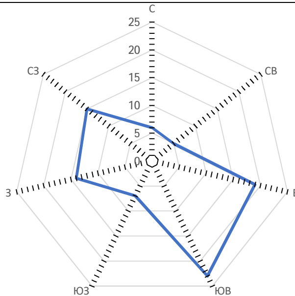
Рисунок 3 – Среднегодовая роза ветров
